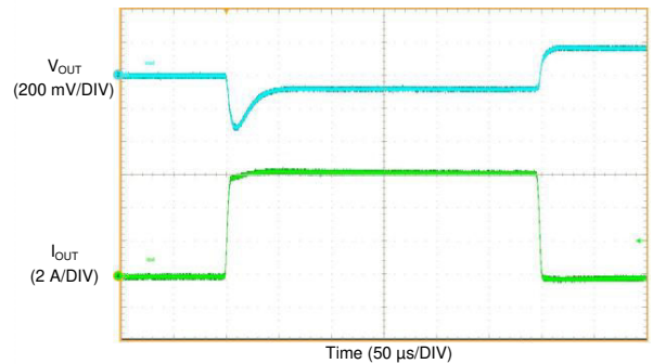
图 9-42. LMQ61460 负载瞬态
