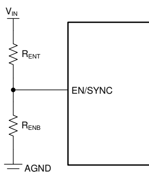
图 8-1. V_{IN} SYNC 使用 EN 引脚
