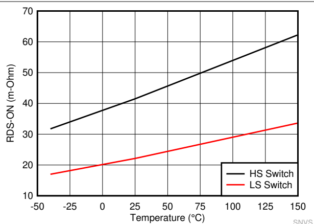
图 7-6. 高侧和低侧开关 R_{DS-ON}
