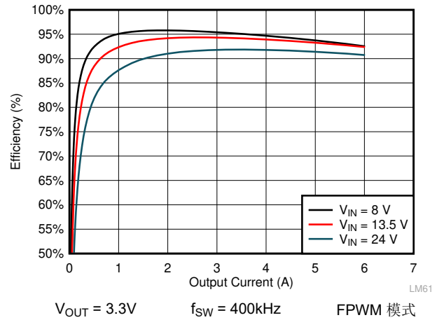
图 9-6. LMQ61460 效率
