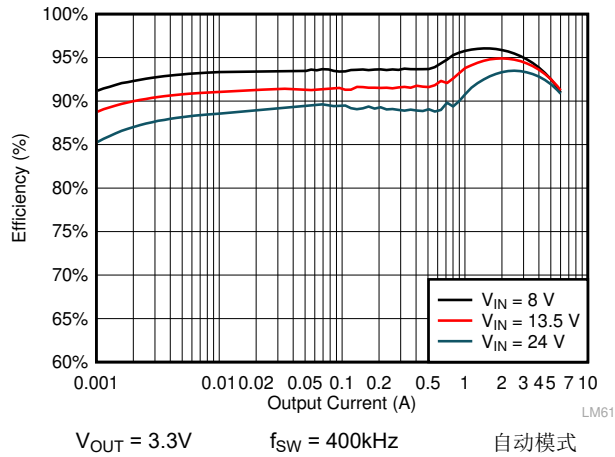
图 9-5. LMQ61460 效率
