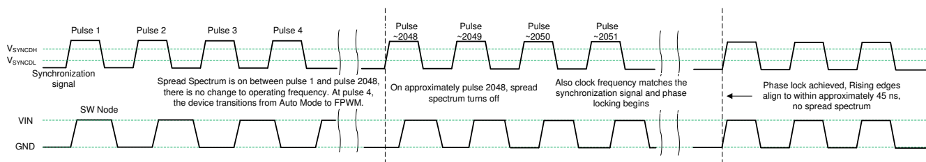
图 8-5. 同步过程
