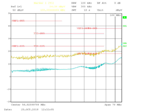
图 9-47. 传导 EMI 与 CISPR25 限值 (黄色: 峰值信号, 蓝色: 平均信号)
