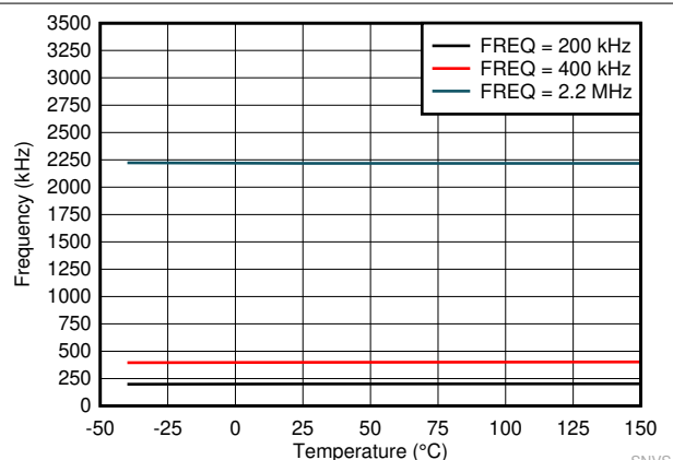
图 7-5. 开关频率
