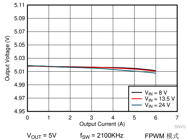
图 9-20. LMQ61460 负载和线性调整率
