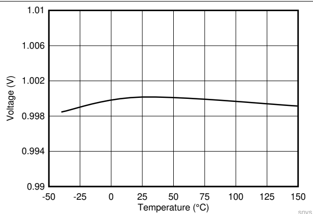
图 7-3. 反馈电压
