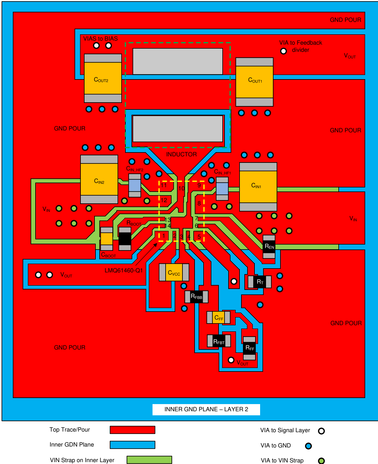
图 11-2. 布局示例
