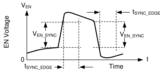
图 8-3. 典型 SYNC/EN 波形
