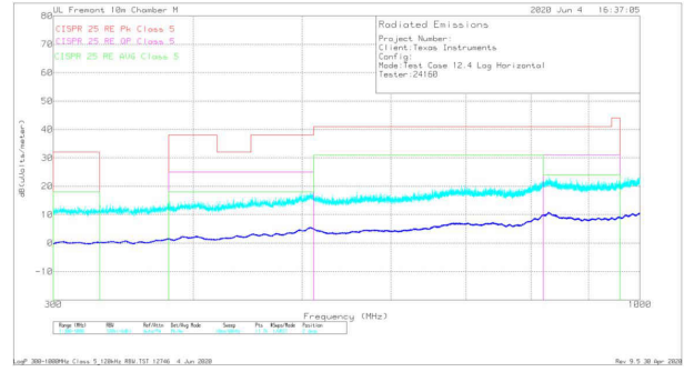
图 9-60. 辐射 EMI 对数水平与 CISPR25 限值
