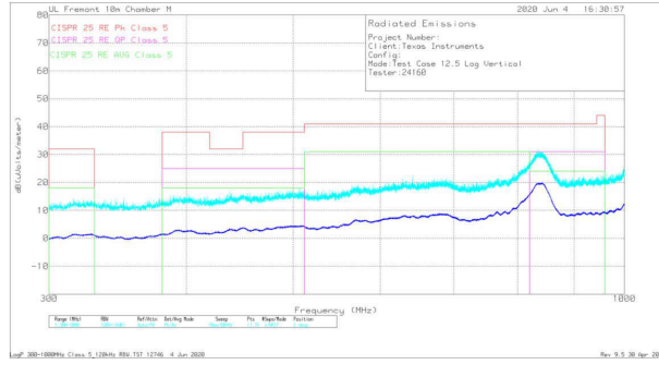
图 9-59. 辐射 EMI 对数垂直与 CISPR25 限值
