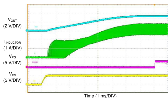
图 9-31. LMQ61460 在 50mA 负载下启动
