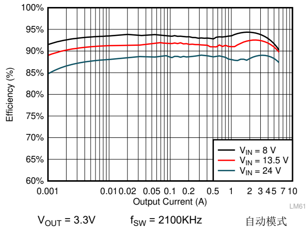
图 9-7. LMQ61460 效率
