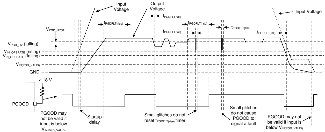
图 8-6. PGOOD 时序图 (不包括 OV 事件)
