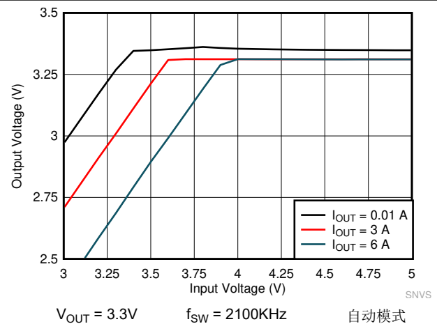
图 9-22. LMQ61460 压降曲线
