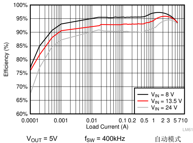
图 9-9. LMQ61460 效率
