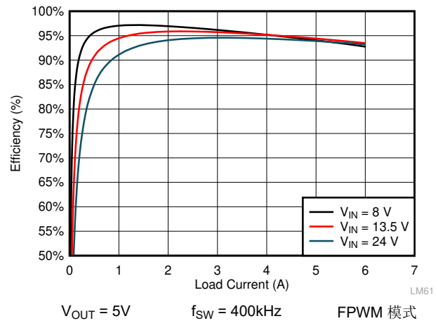
图 9-10. LMQ61460 效率
