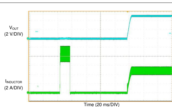
图 8-14. 短路恢复
