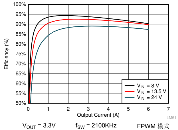
图 9-8. LMQ61460 效率
