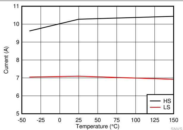
图 7-4. LMQ61460 高侧和低侧电流限制
