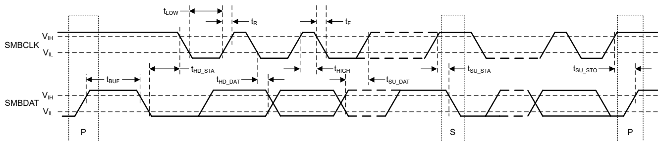
图 6-1. SMBus 时序图
