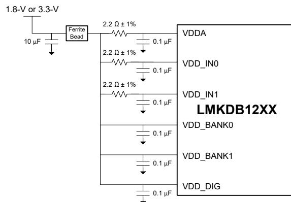
图 10-5. LMKDB12XX 多路复用器的电源建议
