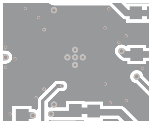
图 10-17. LMKDB1102 布局示例 - 底层
