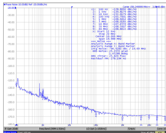
图 10-2. 156.25MHz 下的输入源 (12kHz - 20MHz)
