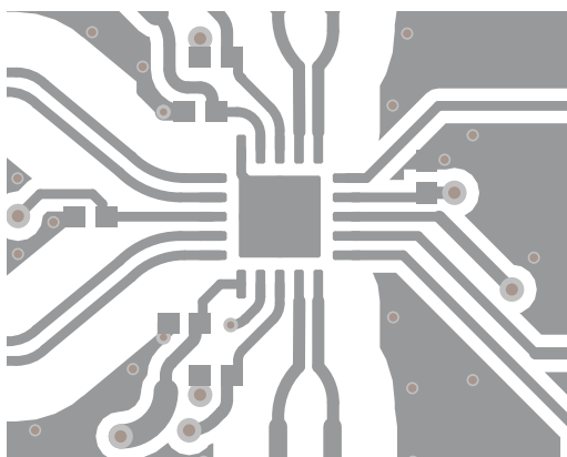
图 10-16. LMKDB1102 布局示例 - 顶层
