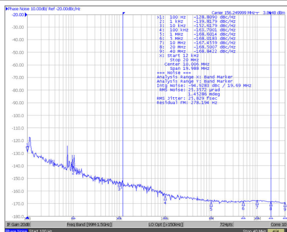
图 6-3. 156.25MHz 下的输入源 (12kHz - 20MHz)
