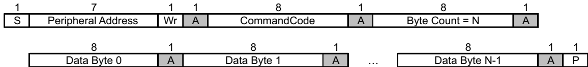
图 8-10. 块写入协议
