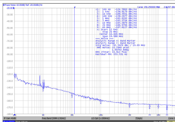
图 6-4. 156.25MHz 下的 LMKDB11xx/120x 相位噪声/输出抖动 (12kHz - 20MHz)
