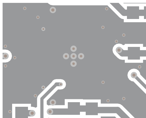
图 10-15. LMKDB1202 布局示例 - 底层
