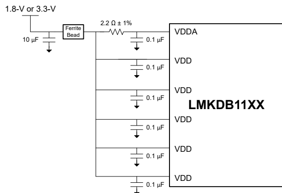
图 10-4. LMKDB11XX 缓冲器的电源建议
