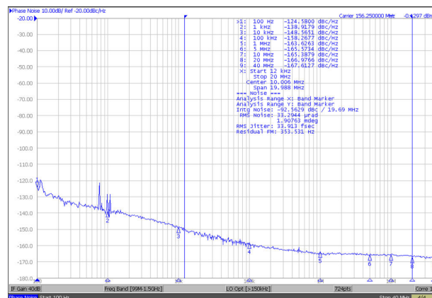
请参阅“图注”表中的注释 1 和注释 2 图 10-3. 156.25MHz 下的 LMKDB11xx/120x 相位噪声/输出抖动 (12kHz - 20MHz)
