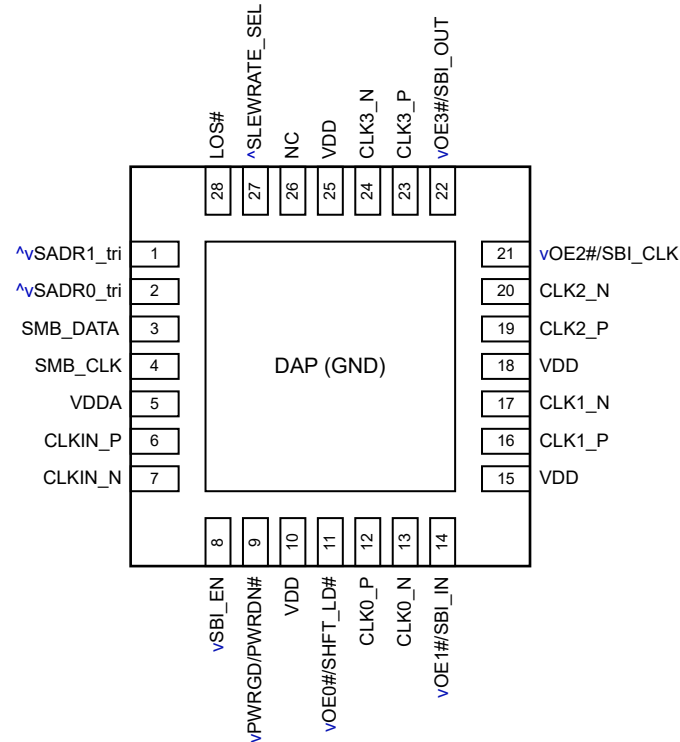
图 5-3. LMKDB1104 4mm x 4mm 28 引脚 QFN
