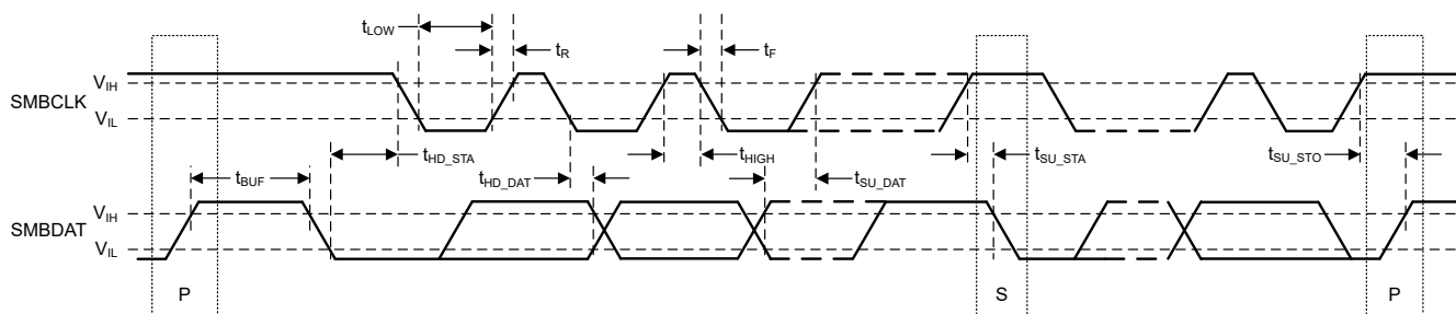
图 6-1. SMBus 时序图
