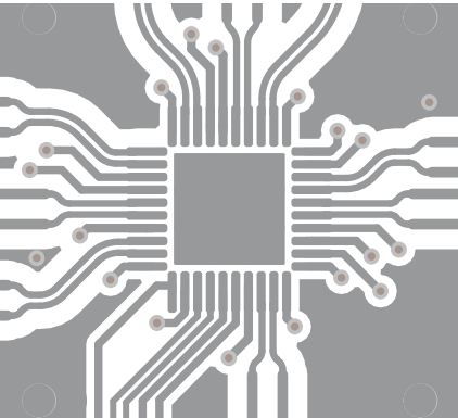
图 10-8. LMKDB1108 布局示例 - 顶层
