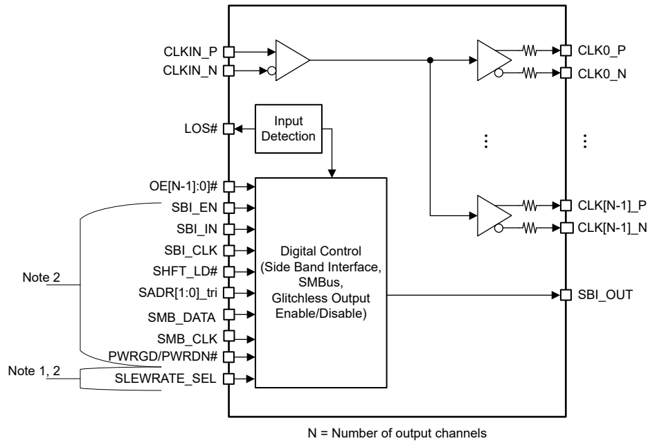
图 8-1. LMKDB11xx 功能方框图
