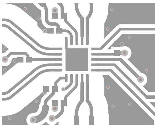
图 10-14. LMKDB1202 布局示例 - 顶层
