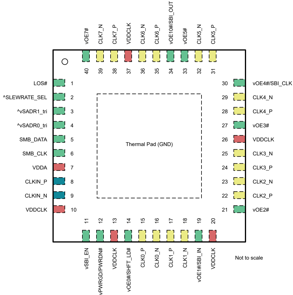
图 5-2. LMKDB1108 和 LMKDB1108FS 5mm x 5mm VQFN 封装 40 引脚 顶视图
