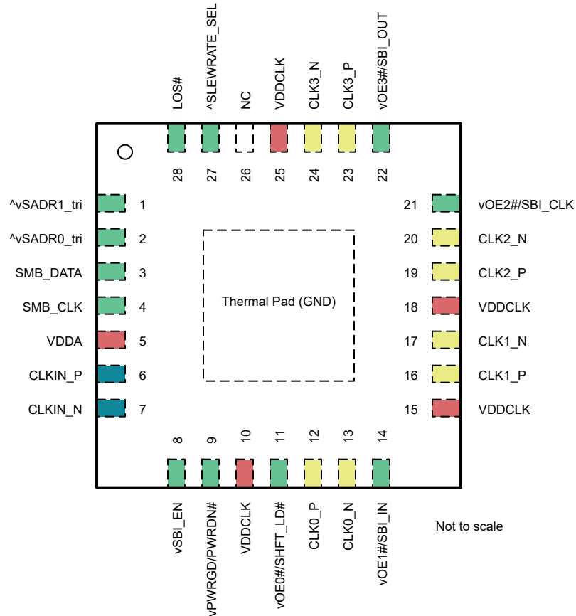
图 5-3. LMKDB1104 和 LMKDB1104FS 4mm x 4mm VQFN 封装 28 引脚 顶视图
