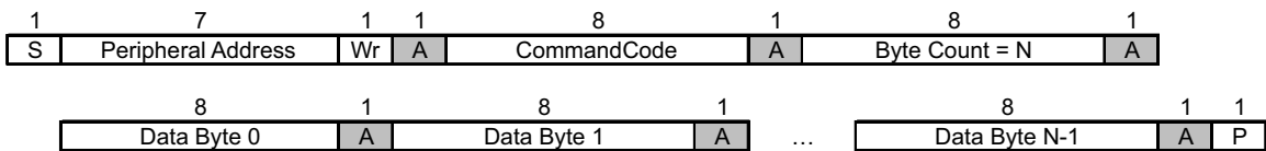
图 8-10. 块写入协议
