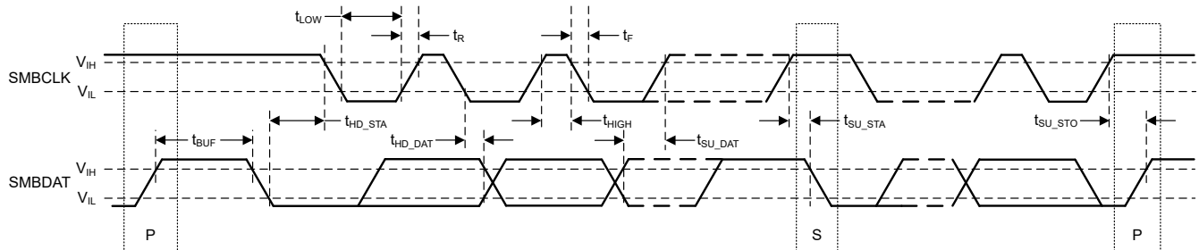
图 6-1. SMBus 时序图
