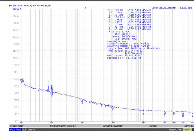
图 6-4. 156.25MHz 下的 LMKDB11xx 相位噪声/输出抖动 (12kHz - 20MHz)
