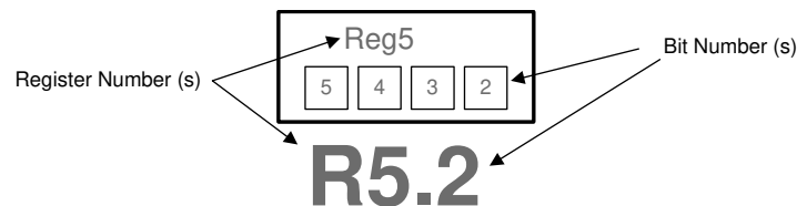
图 8-1. LMK61E07 Register Reference Format
