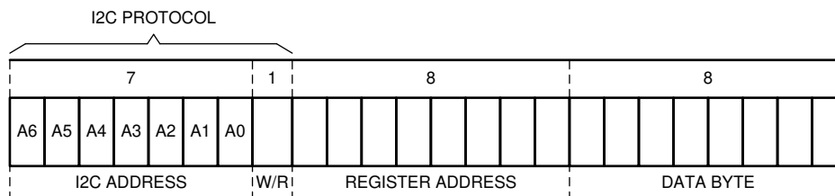
图 8-6. I 2 C Register Structure
