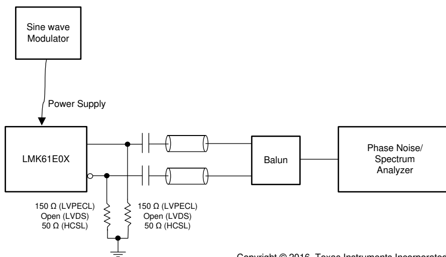
图 7-7. PSRR Test Setup
