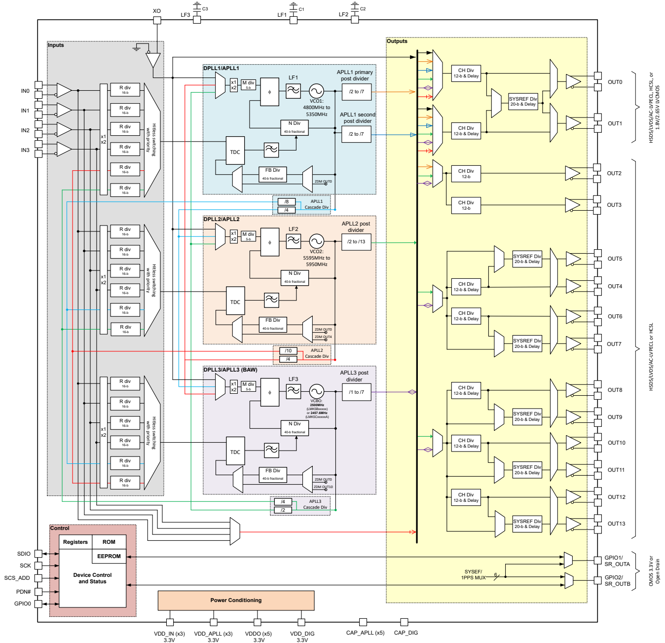
图 8-1. LMK5C33414AS1 顶层方框图
