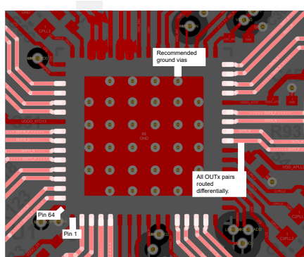
图 9-5. LMK5C33414AS1 的 PCB 布局示例，顶层
