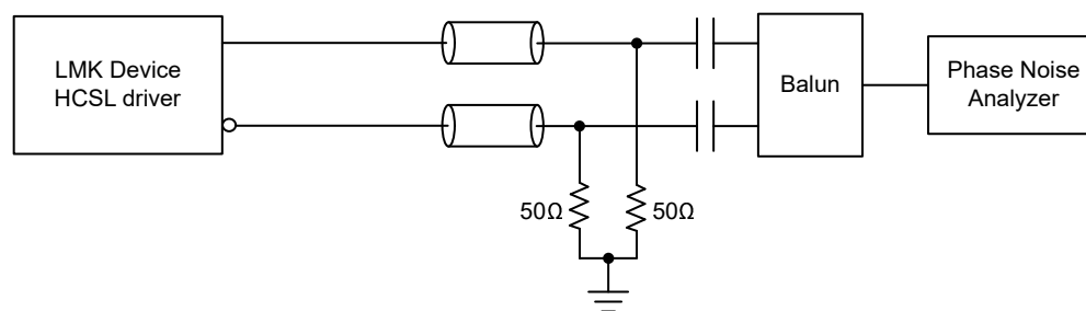
图 7-8. HCSL 输出相域测试配置
