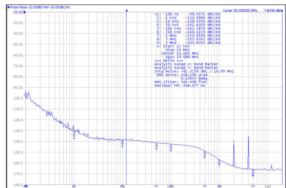
图 6-19. APLL1 的 50MHz HSDS 输出
