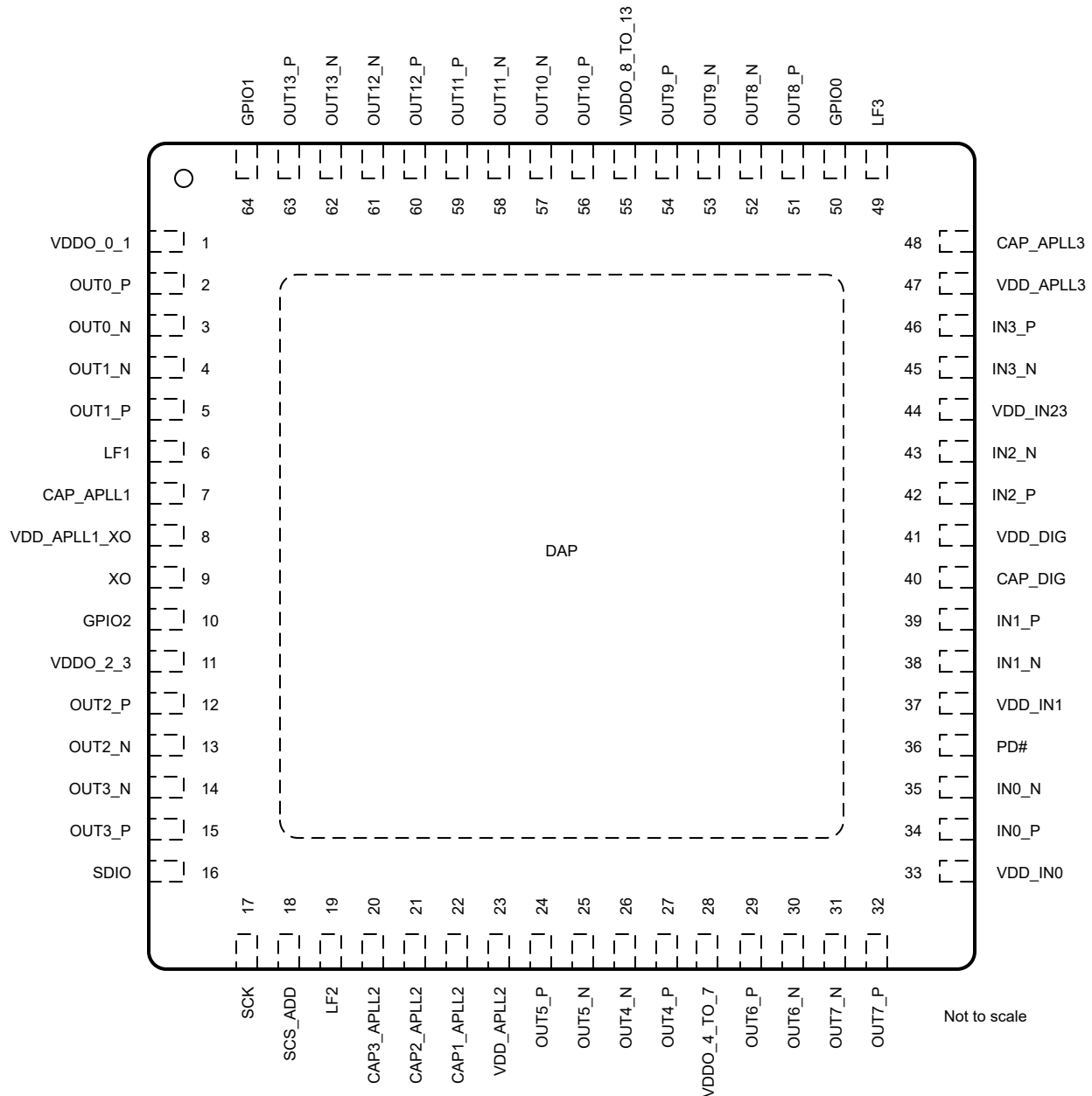
图 5-1. LMK5C33414AS1 RGC 封装 64 引脚 VQFN 顶视图
