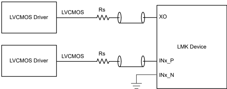
图 8-10. 单端 LVCMOS ( 1.8V、2.5V、3.3V ) 至基准 (INx_P) 或 XO 输入 (XO)
