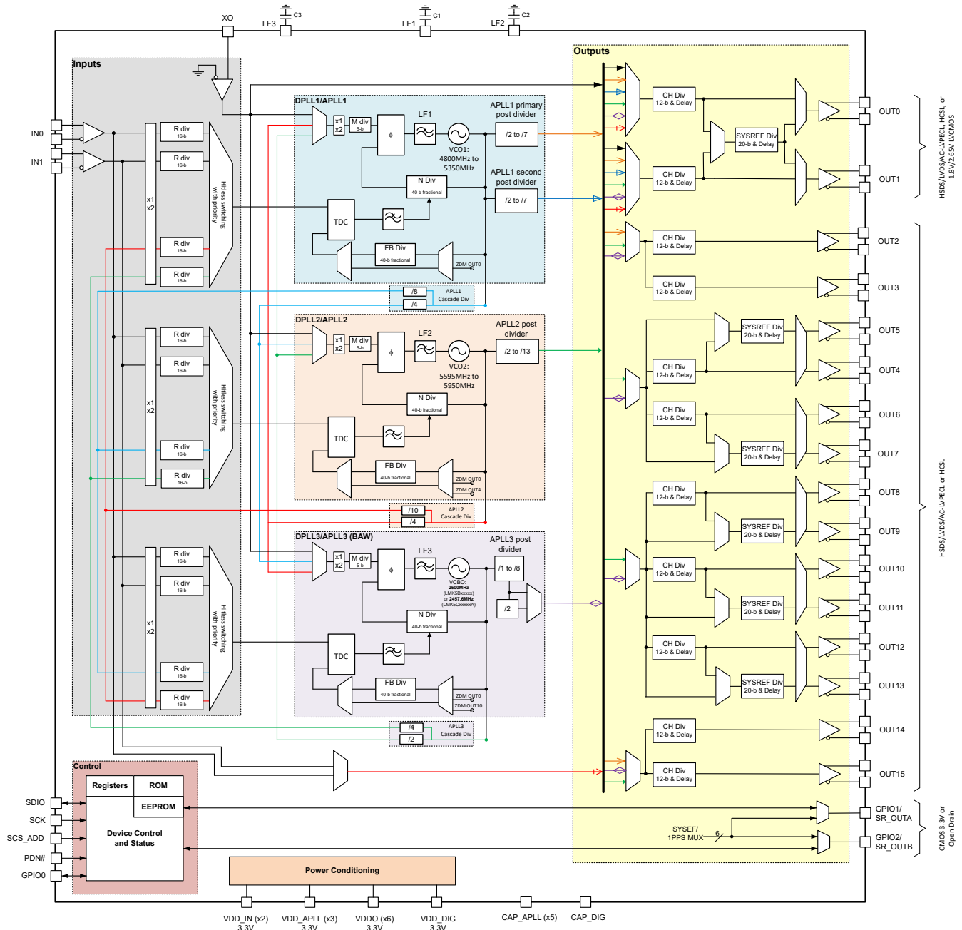
图 8-1. LMK5C33216AS1 顶层方框图
