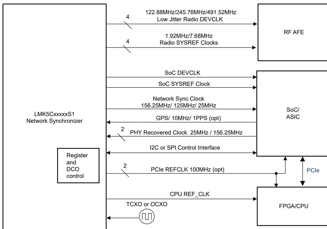
LMK5C33216AS1 典型系统方框图
