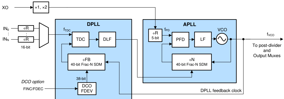
图 8-23. PLL 架构
