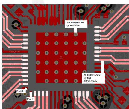
图 9-5. LMK5C33216AS1 的 PCB 布局示例，顶层
