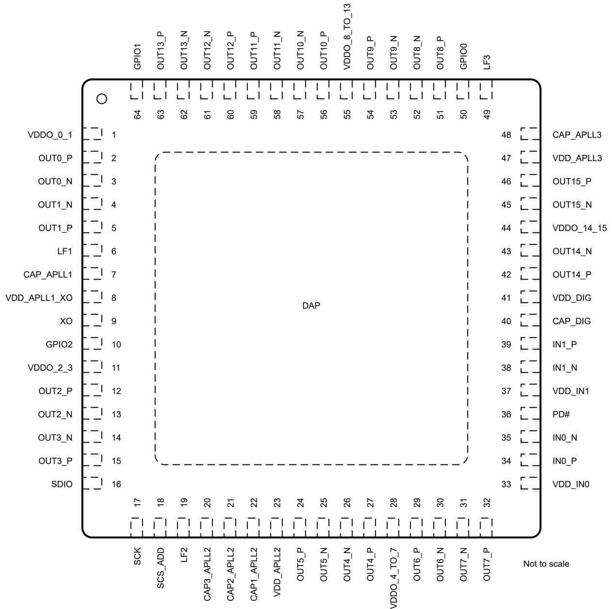
图 5-1. LMK5C33216AS1 RGC 封装 64 引脚 VQFN 顶视图
