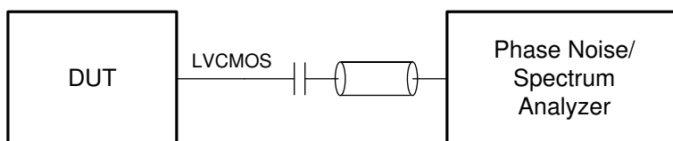
图 8-4. LVC MOS Output Phase Noise Test Configuration
