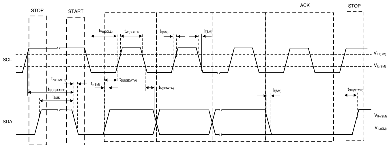
图 7-4. I²C Timing Diagram
