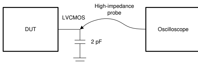
图 8-3. LVC MOS Output DC Test Configuration
