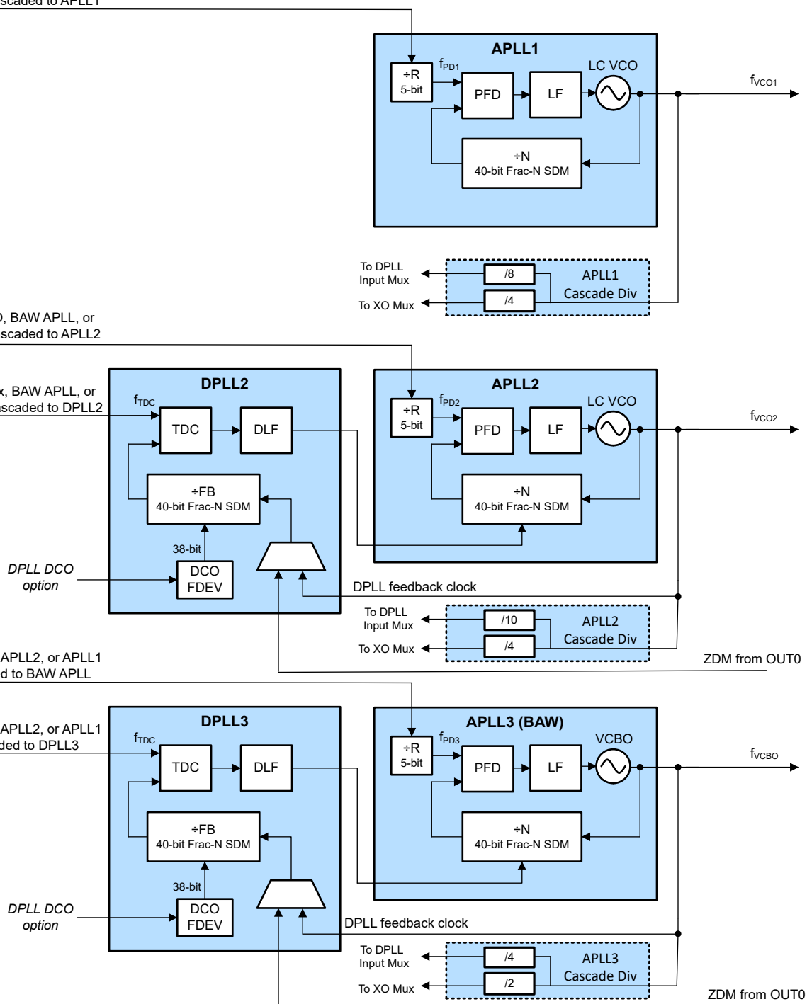
图 8-2. PLL 架构
