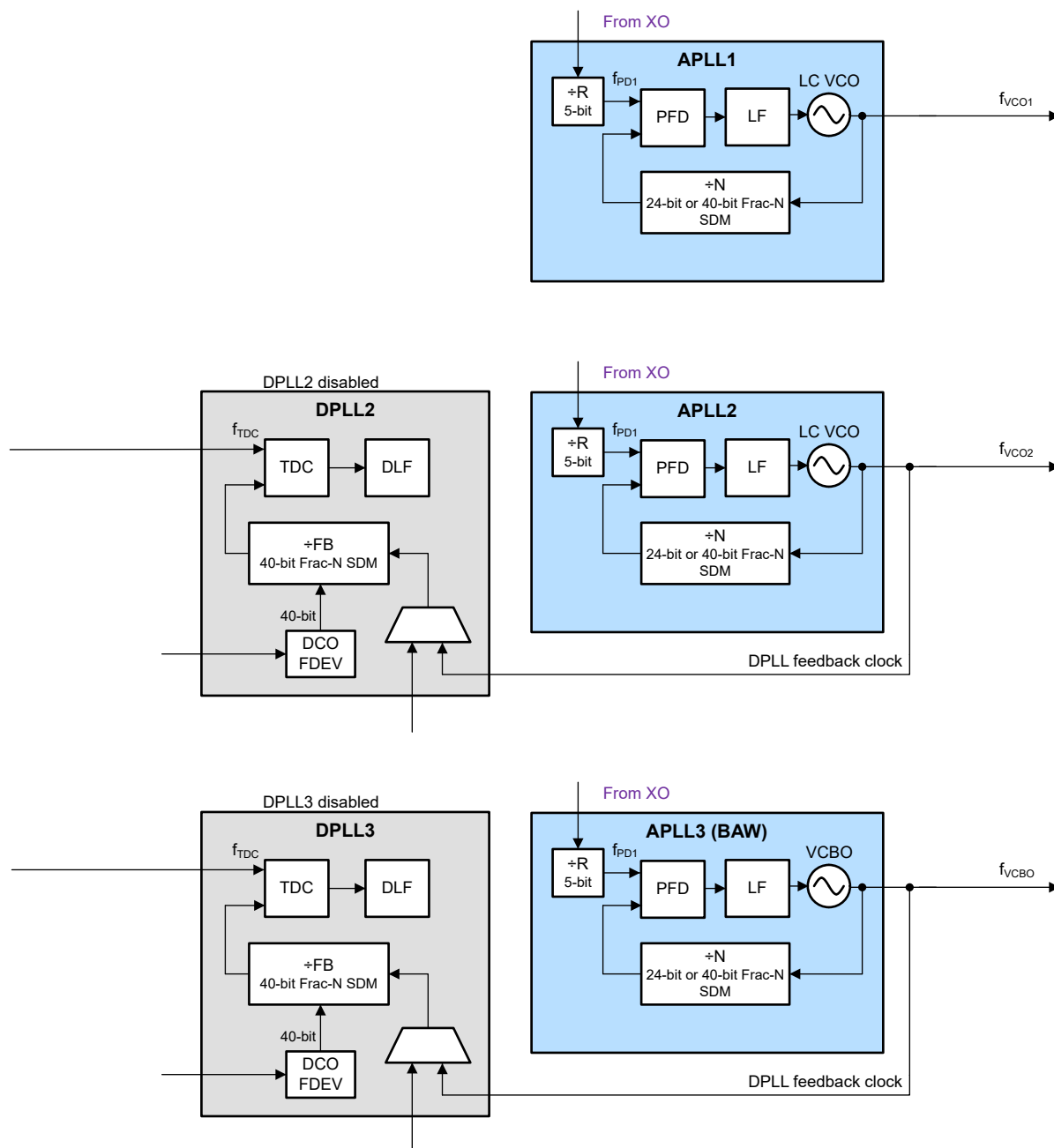
图 8-7. 仅 APLL 独立模式
