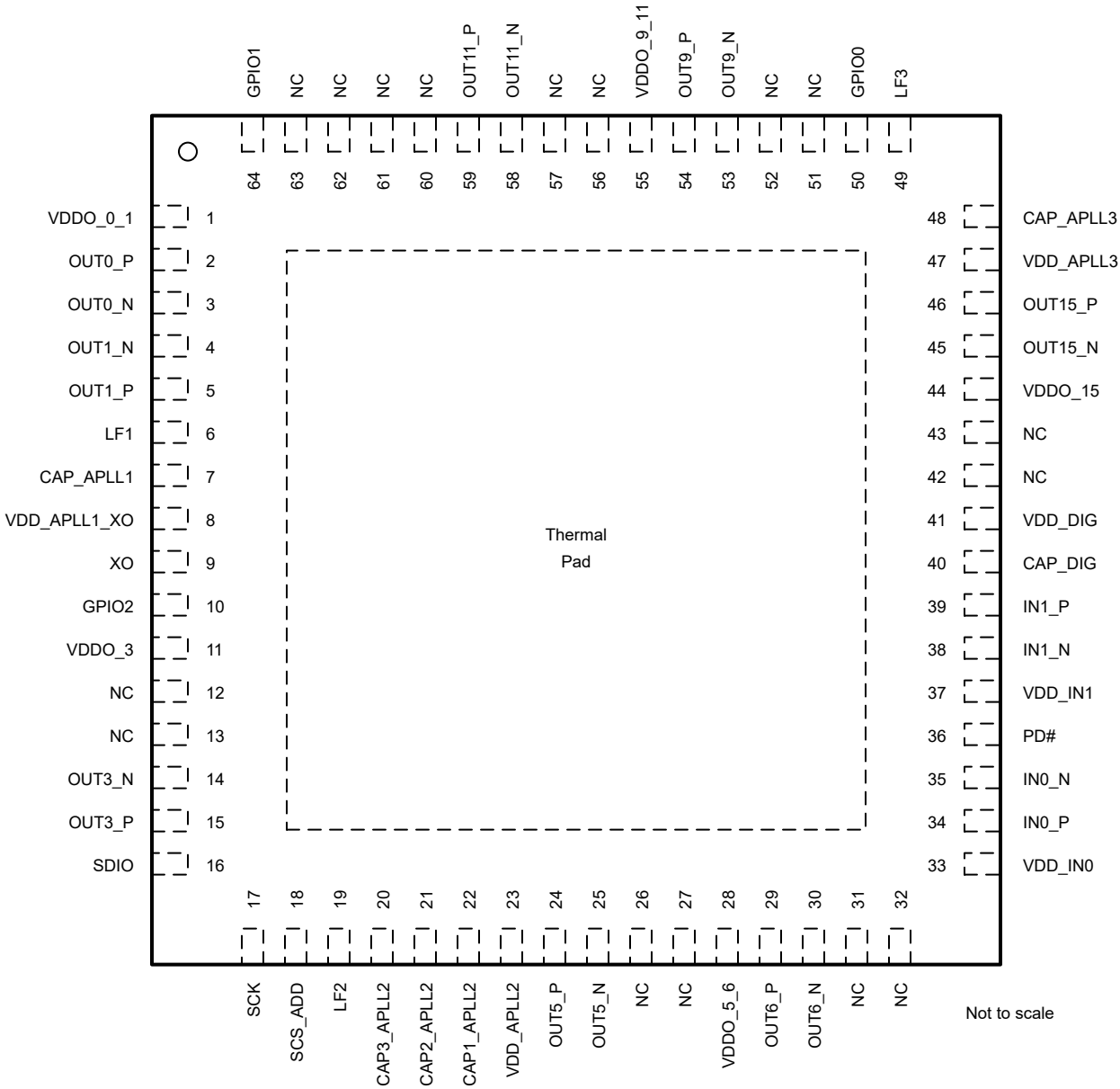
图 5-1. LMK5C23208A RGC 封装 64 引脚 VQFN 顶视图
