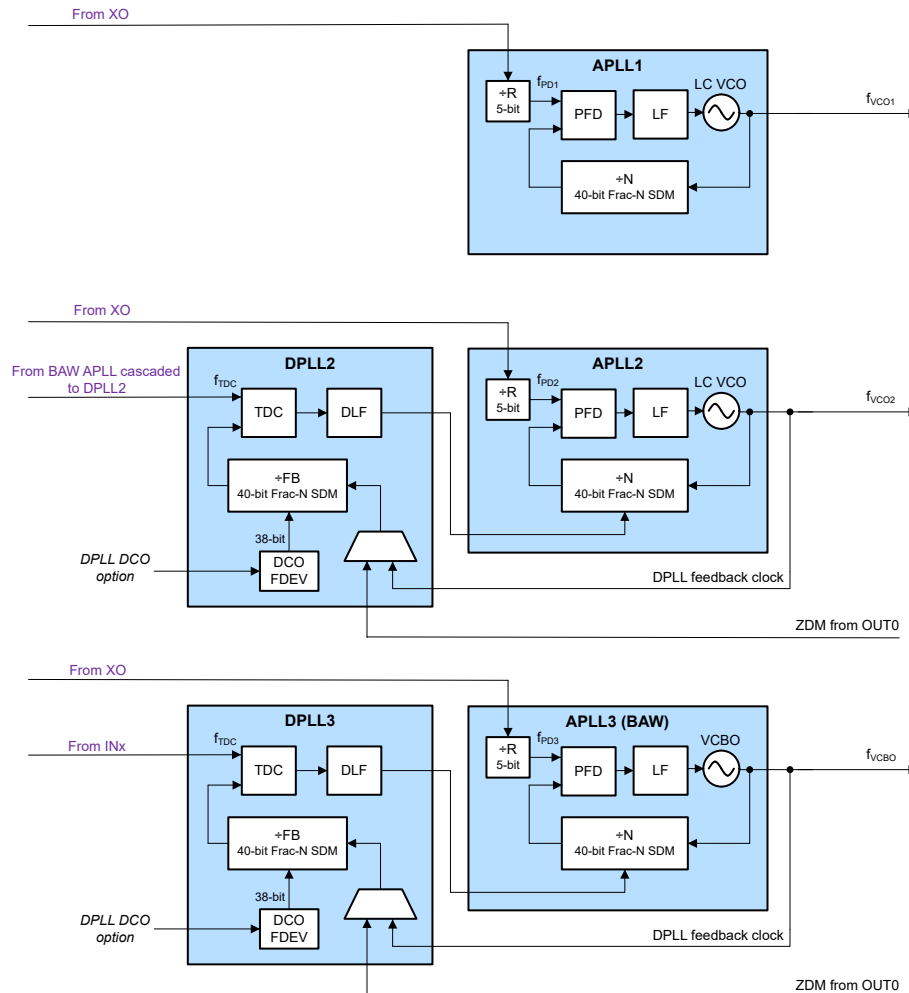
图 8-4. DPLL 级联模式
