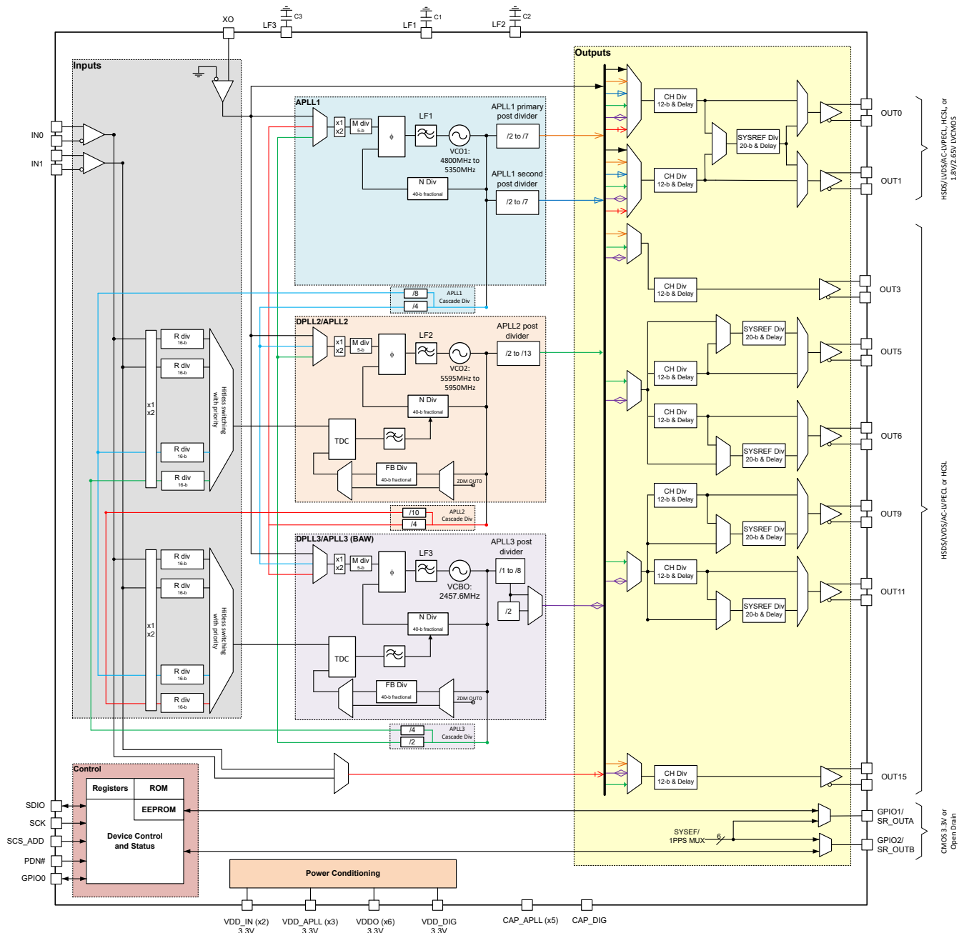
图 8-1. LMK5C23208A 顶层方框图
