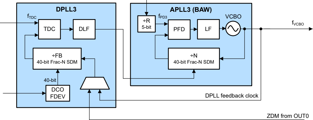
图 8-6. 禁用 DPLL 的 APLL 级联示例
