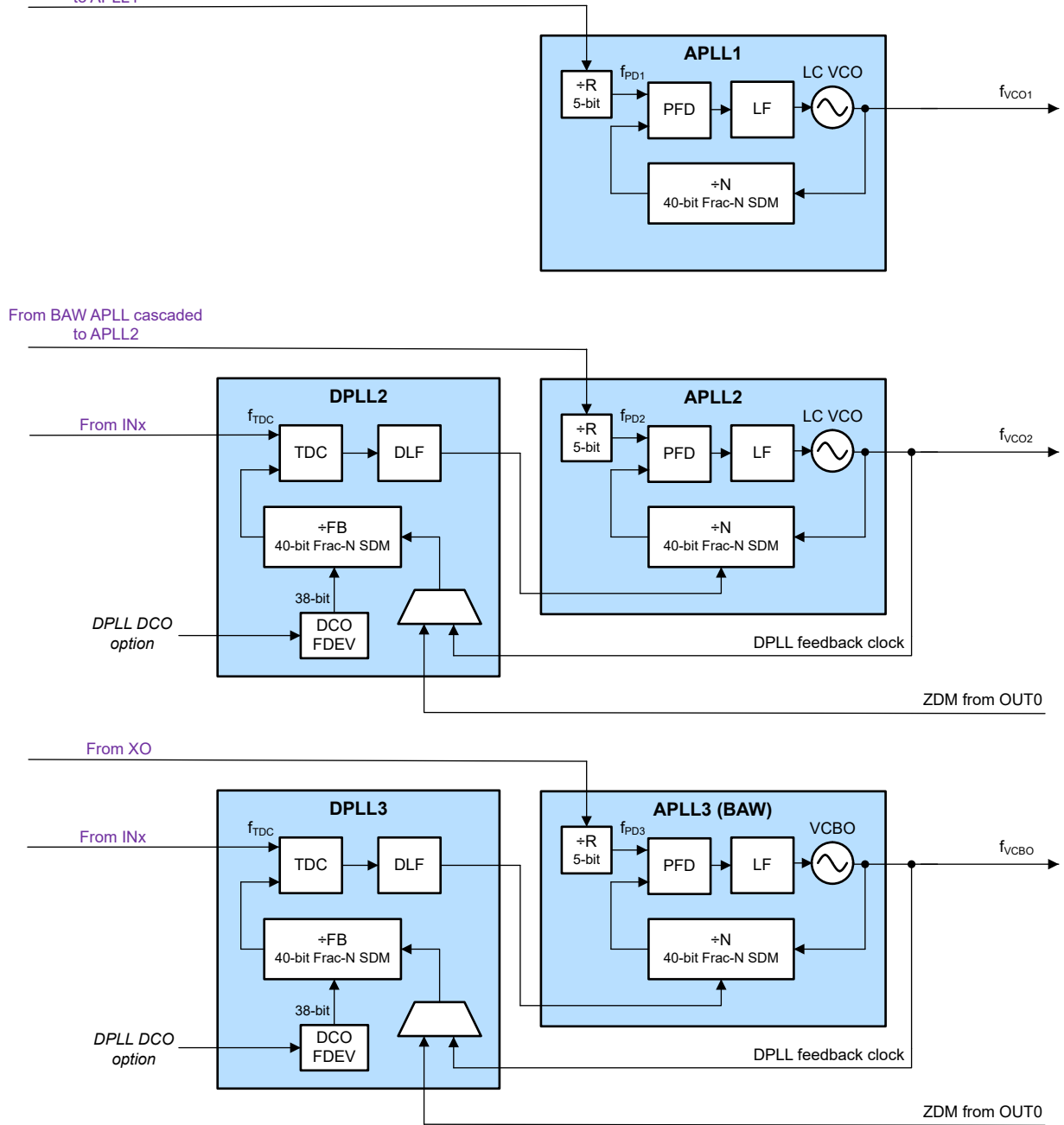
图 8-5. 启用 DPLL 的 APLL 级联示例
