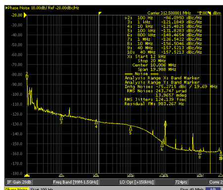
图 6-12. APPL2 的 312.5MHz HSDS 输出
