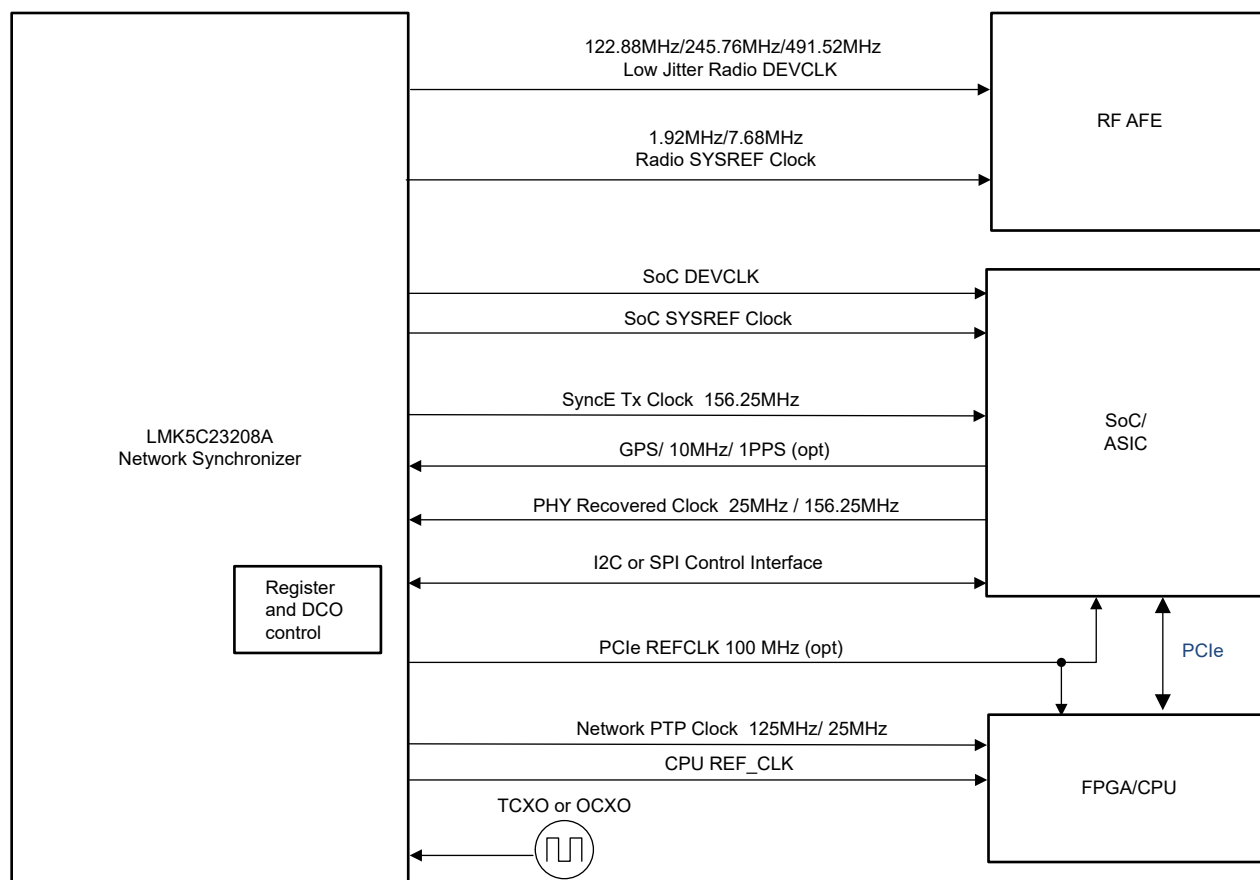
LMK5C23208A 典型系统方框图
