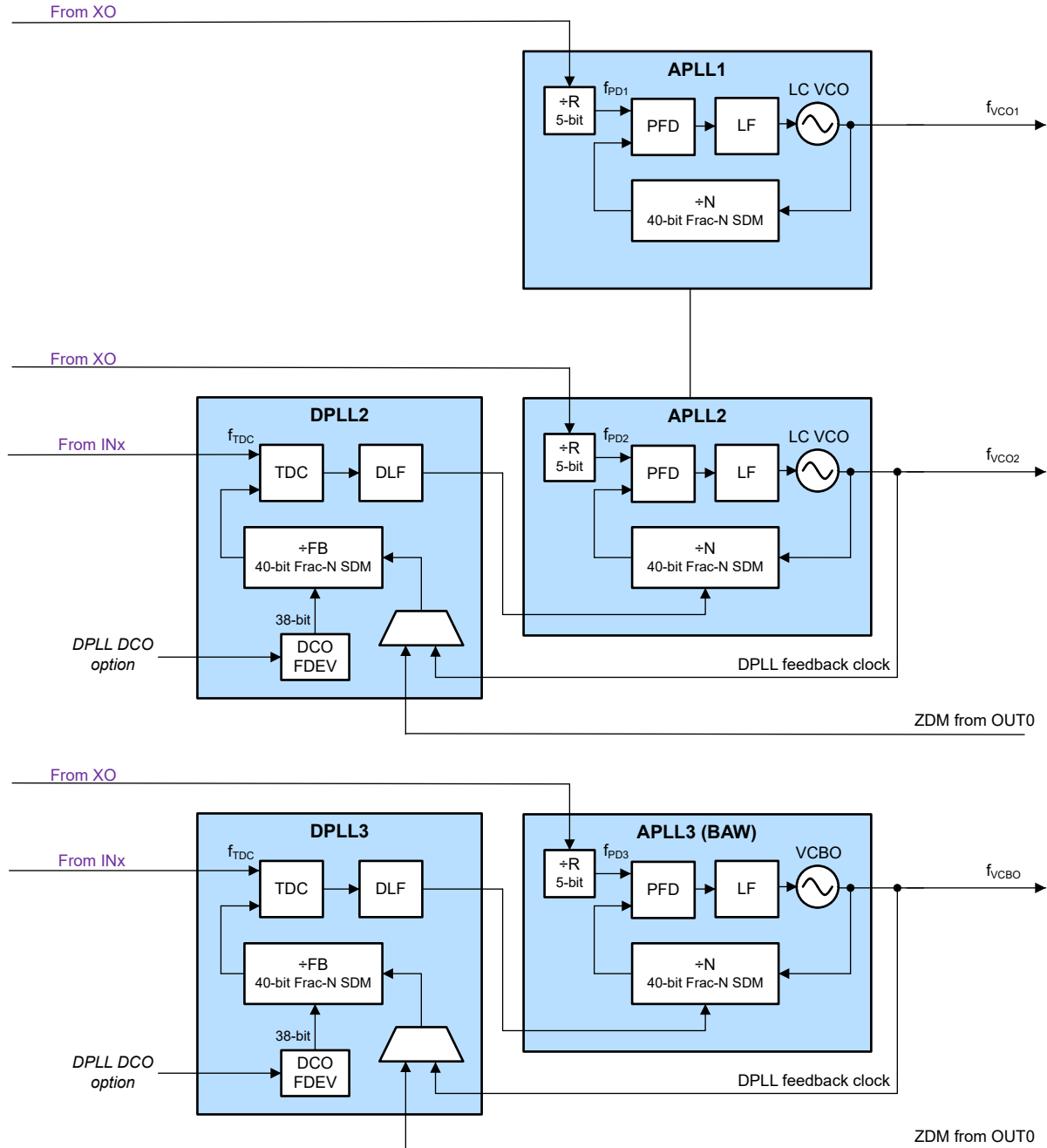
图 8-3. DPLL 独立模式
