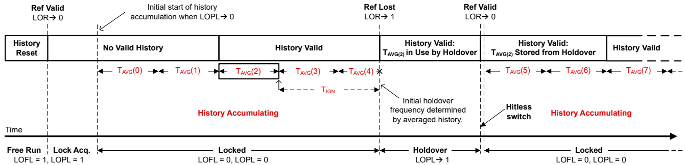
图 7-21. 调优字历史记录窗口
