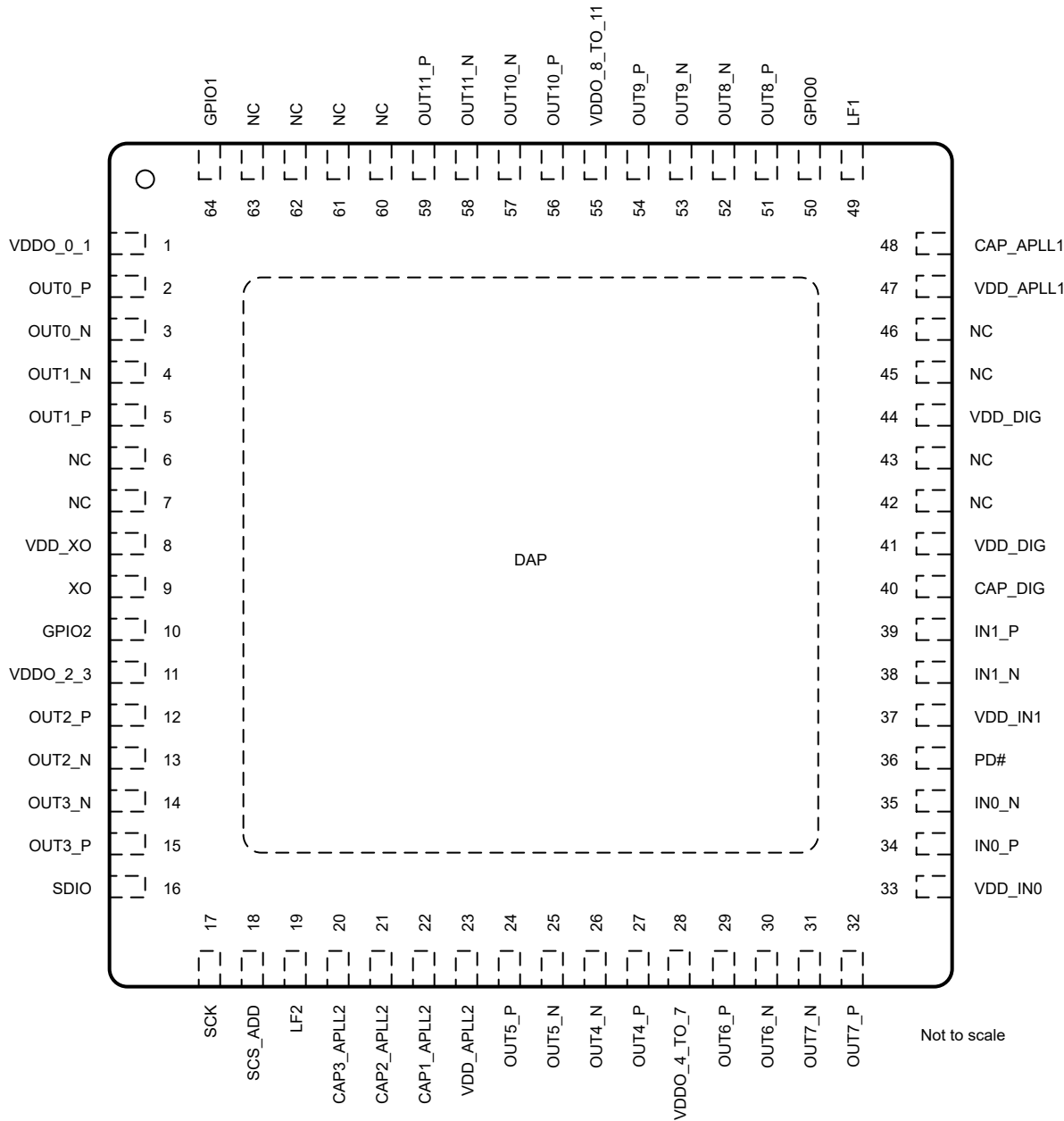
图 4-1. LMK5C22212A RGC 封装 64 引脚 VQFN 顶视图
