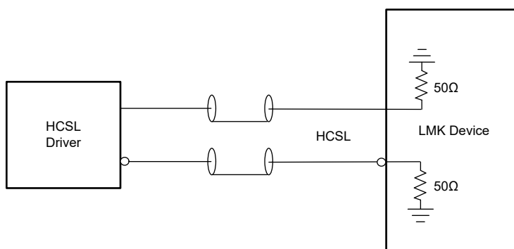
图 7-14. HCSL (负载端接) 至基准 (INx)
