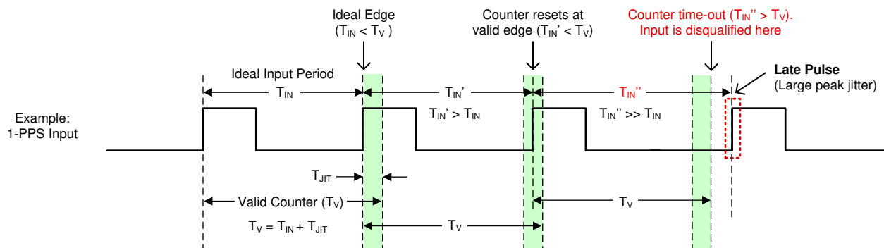
图 7-19. 1PPS 输入窗口检测器示例
