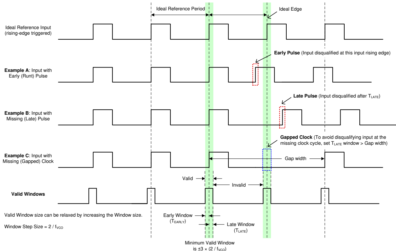
图 7-18. 早期和晚期窗口检测器示例
