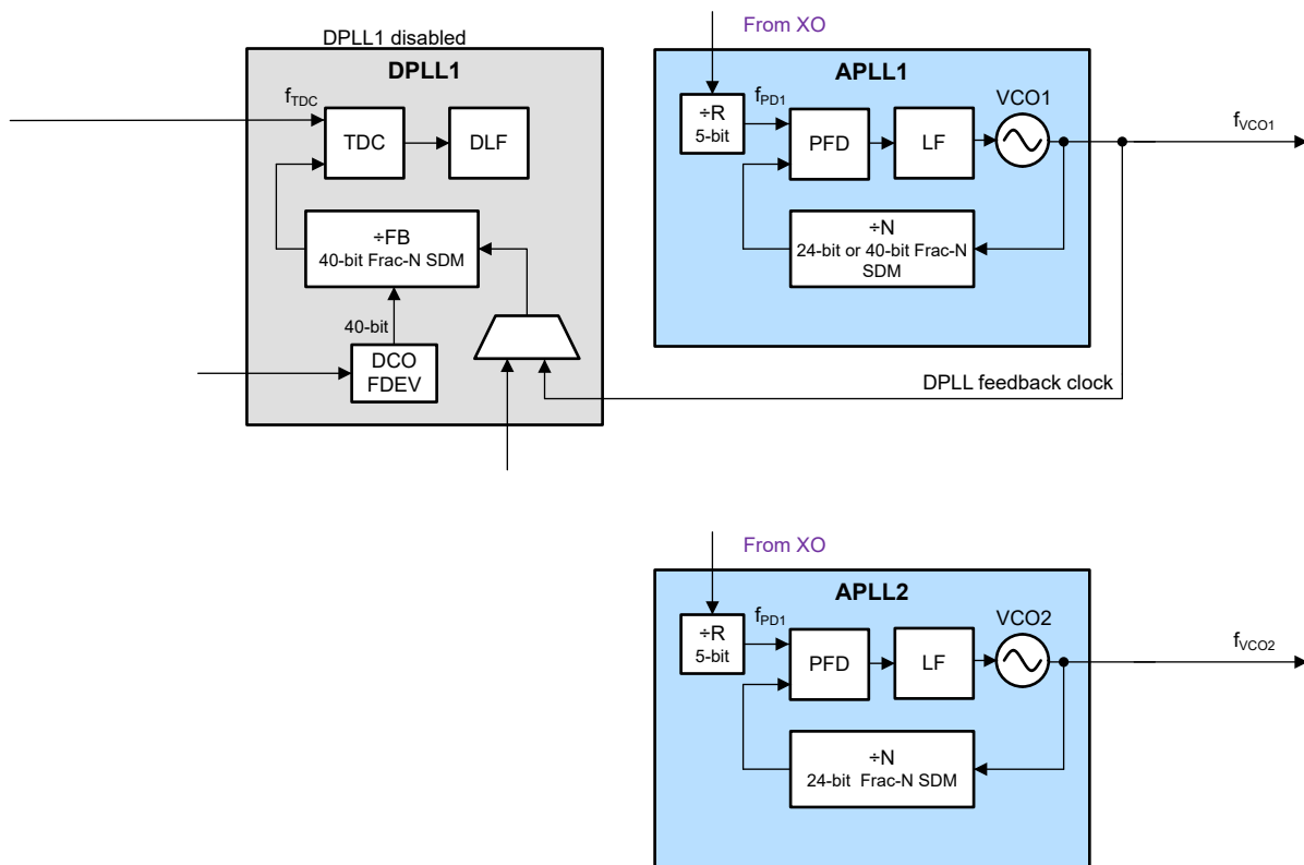
图 7-7. 仅 APLL 独立模式
