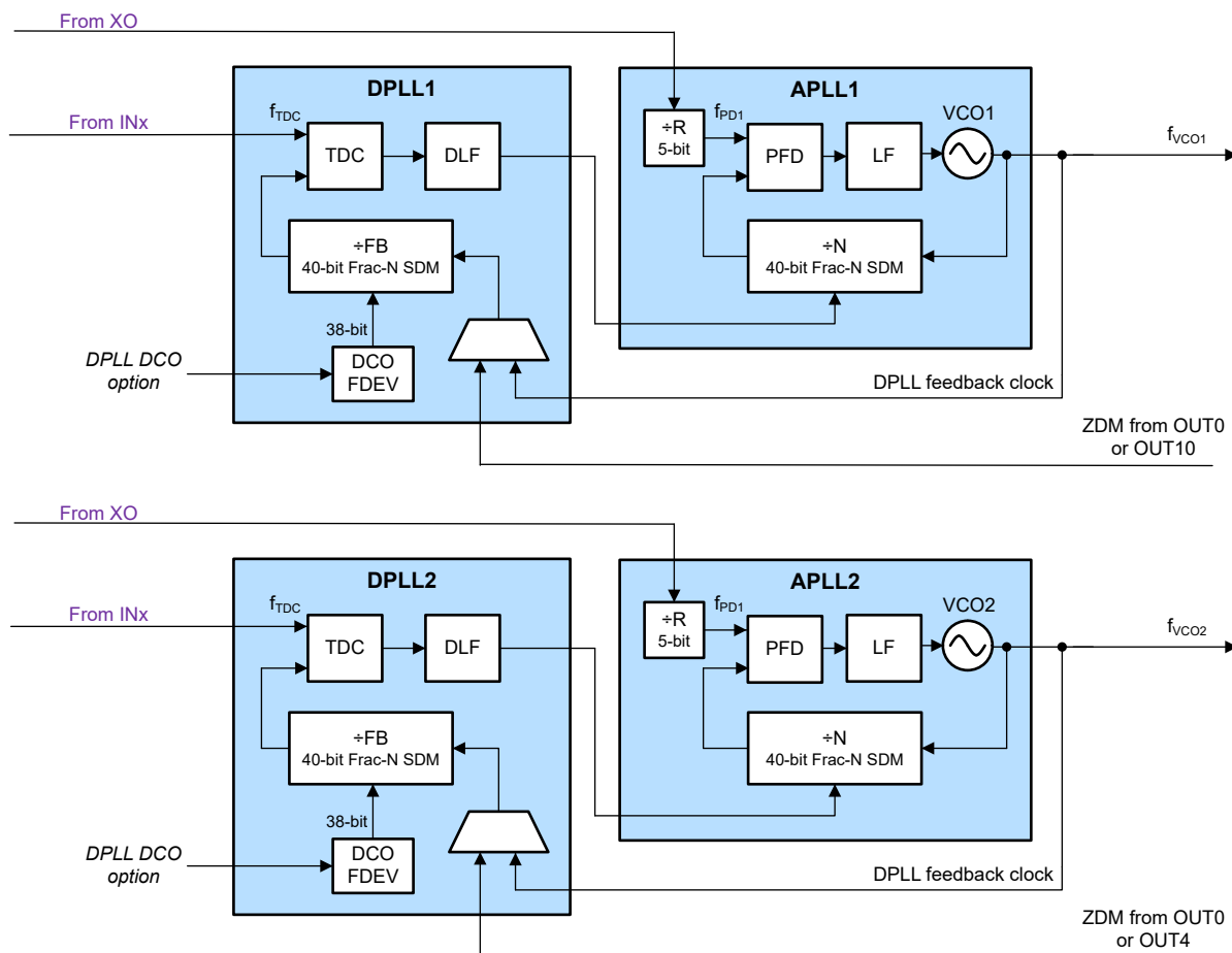
图 7-3. DPLL 操作
