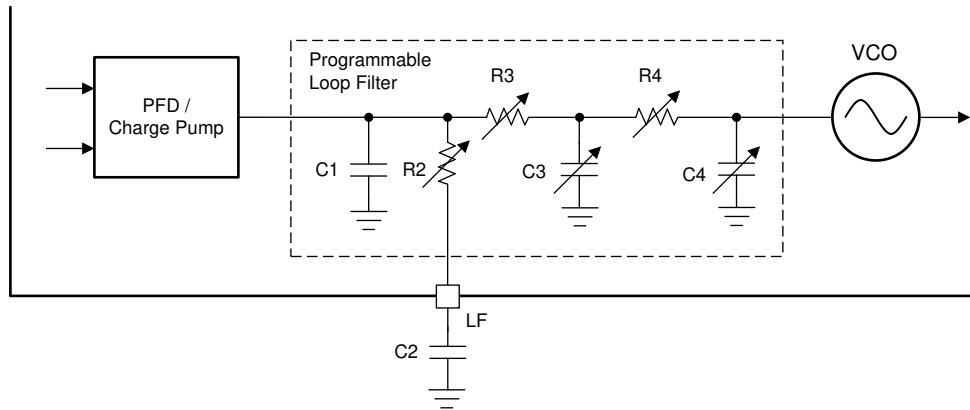
图 7-24. 每个 APLL 的环路滤波器结构
