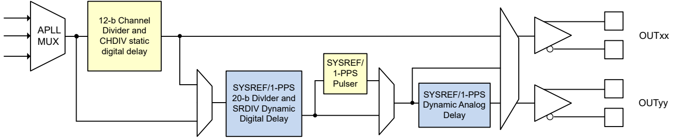
图 7-25. 可编程静态和动态输出延迟
