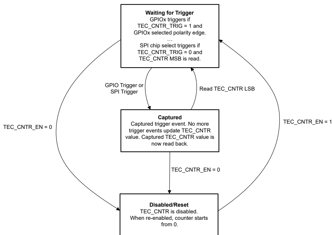
图 7-34. TEC 的状态图
