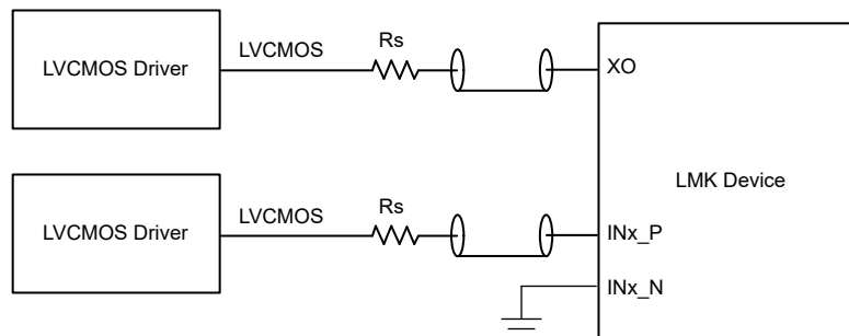
图 7-10. 单端 LVCMOS (1.8V、2.5V、3.3V) 至基准 (INx_P) 或 XO 输入 (XO)
