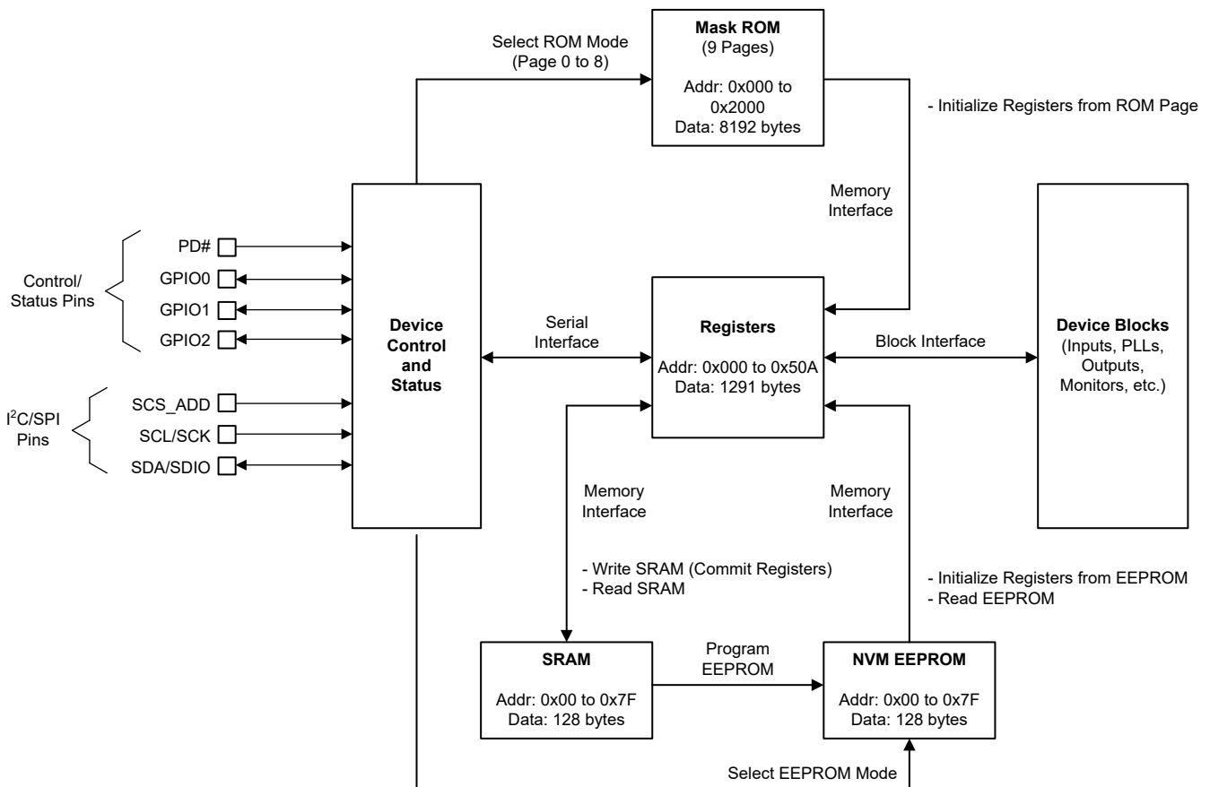
图 7-43. 器件控制、寄存器和存储器接口
