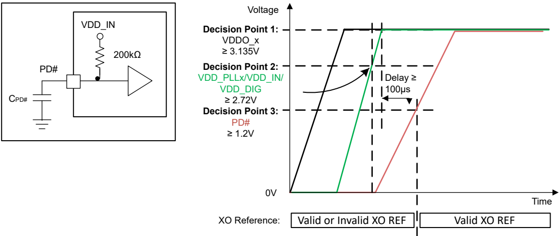
图 8-2. 从双电源轨上电的建议
