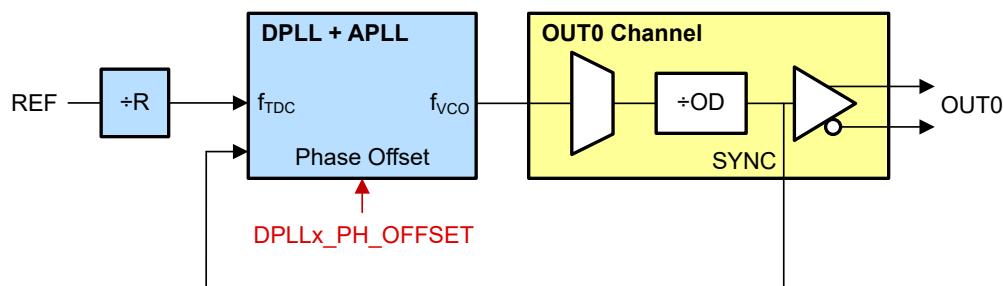
图 7-32. 基准输入和 OUT0 之间的 DPLL ZDM 同步
