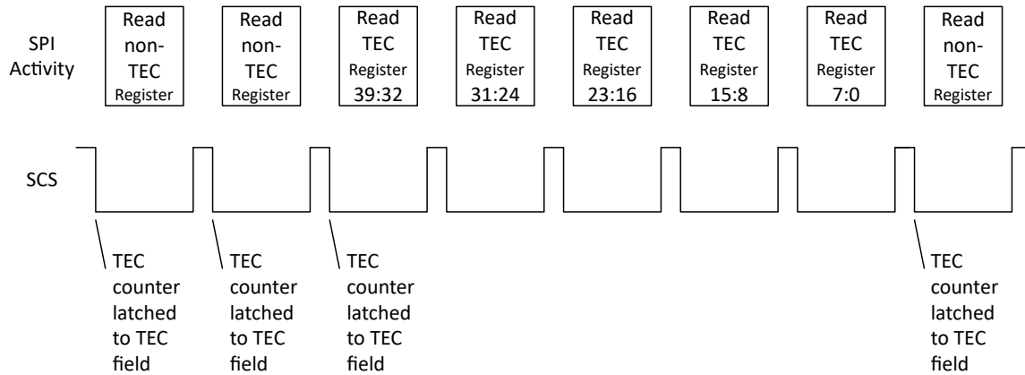
图 7-35. TEC 单字节读取
