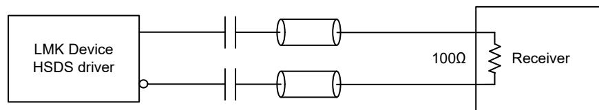
图 7-28. 交流耦合 HSDS 输出端接方法 1
