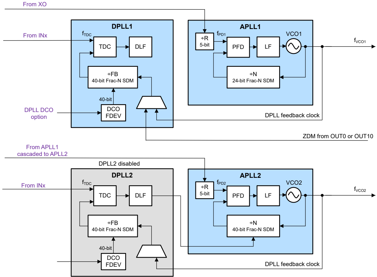
图 7-6. 禁用 DPLL 的 APLL 级联示例
