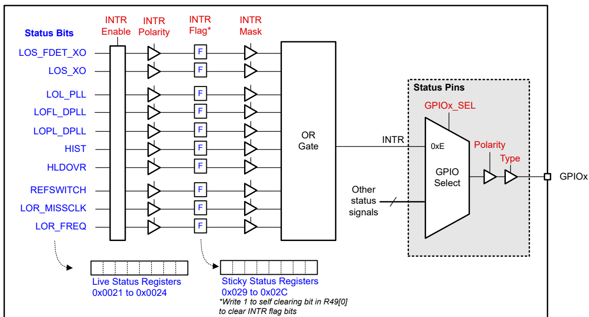
图 7-22. 状态和中断
