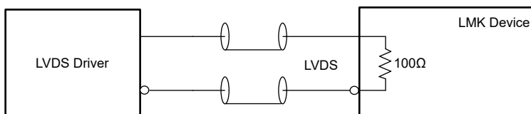
图 7-12. 直流耦合 HSDS/LVDS 至基准 (INx)
