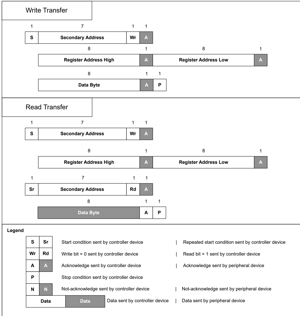
图 7-45. I 2 C 字节写入和读取传输
