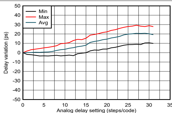
图 5-17. SYSREF/1PPS 延迟线性度与模拟延迟代码 2
