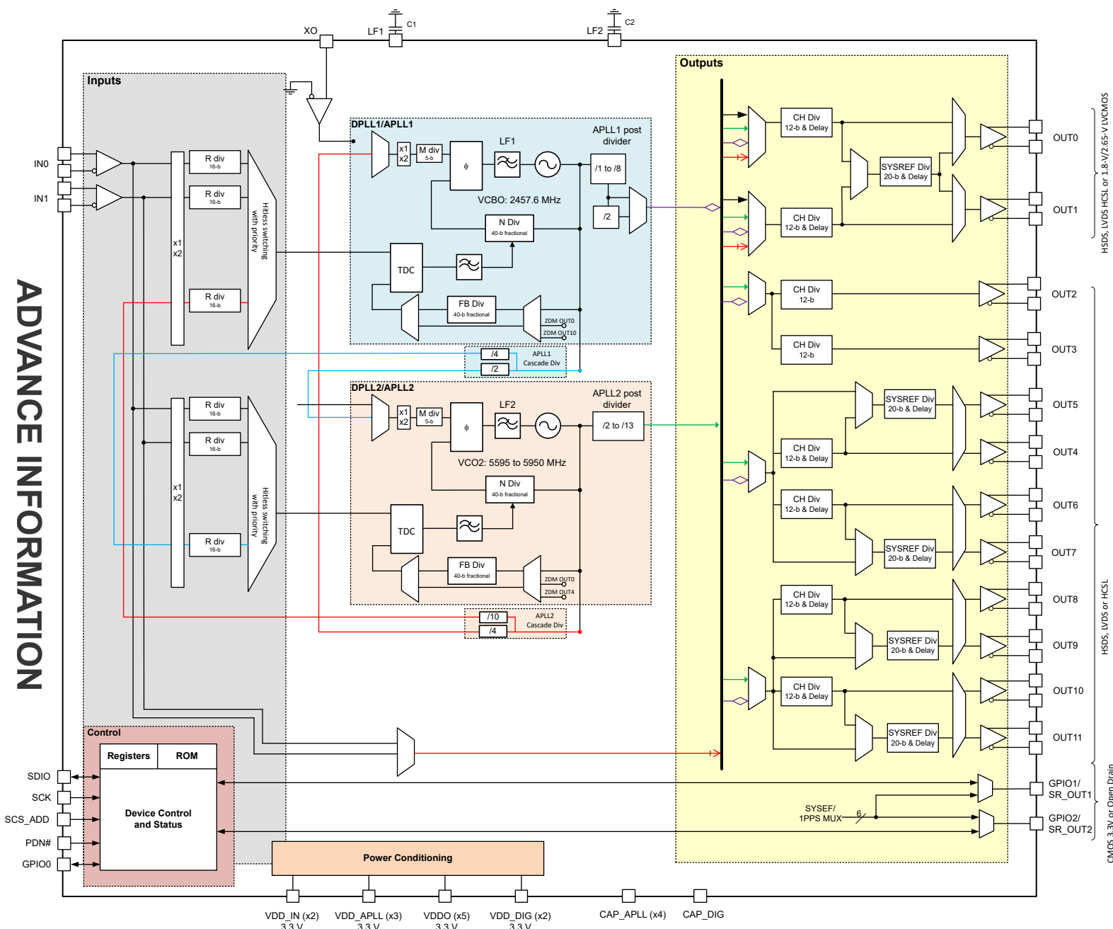
图 7-1. LMK5C22212A 顶层方框图
