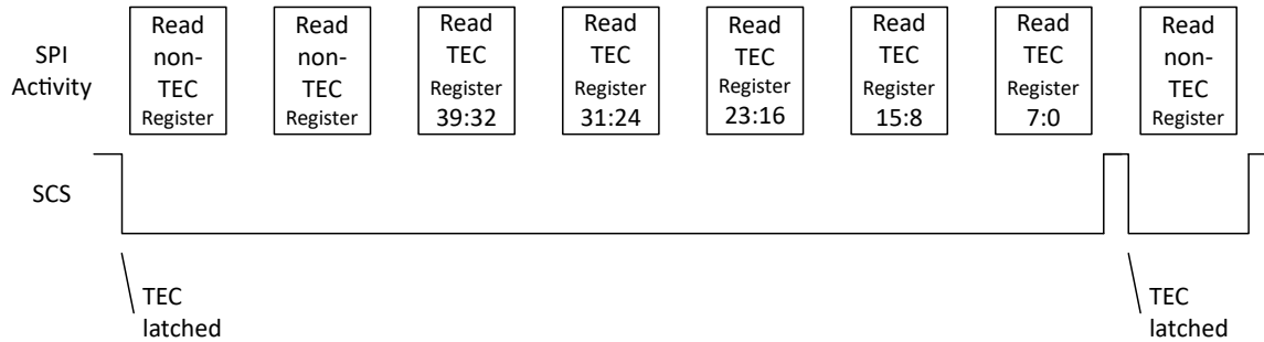
图 7-36. TEC 多字节读取
