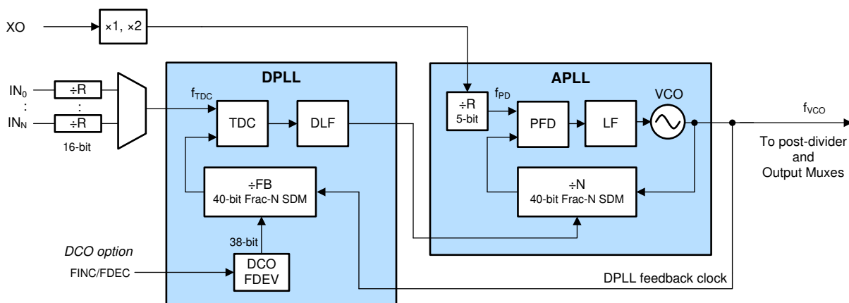
图 7-23. PLL 架构
