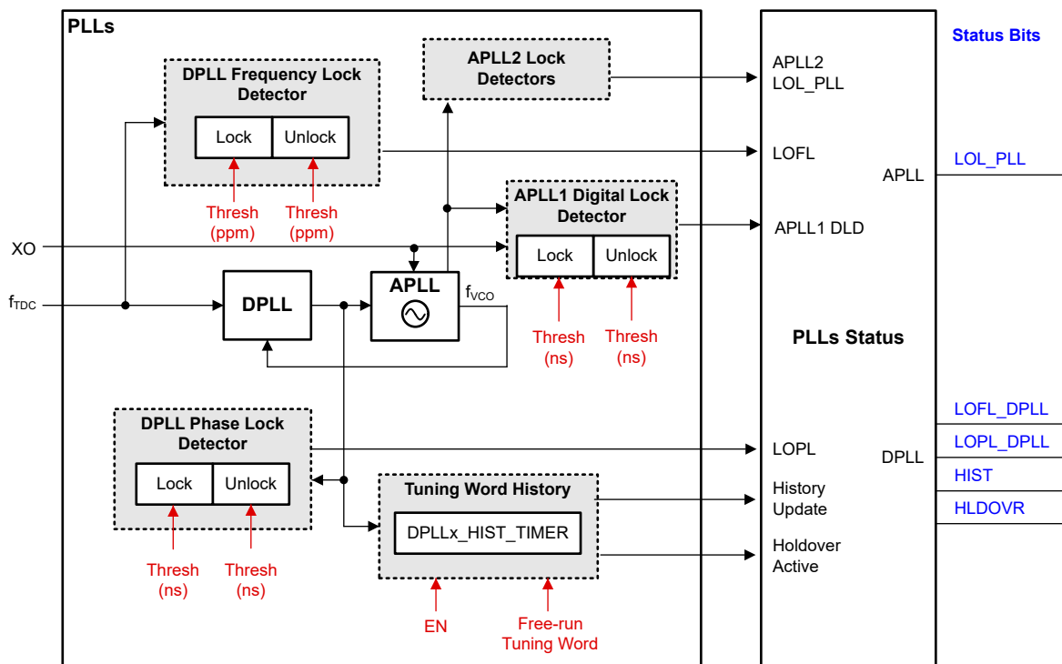
图 7-20. PLL 锁定检测器和历史记录监控器
