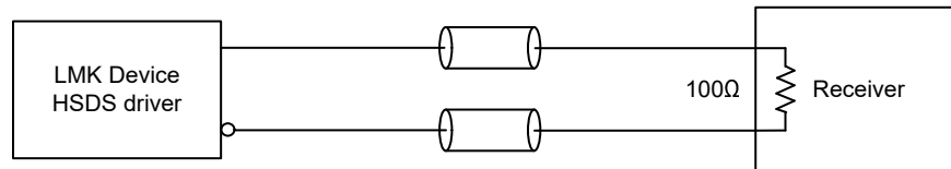
图 7-27. 直流耦合 HSDS/LVDS 输出终端
