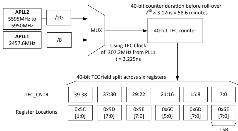
图 7-34 展示了历时计数器函数的状态。
