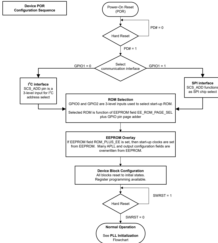
图 7-41. 器件 POR 序列
