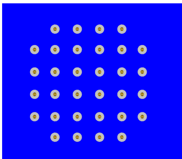
图 8-6. LMK5C22212A 的 PCB 布局示例，底层
