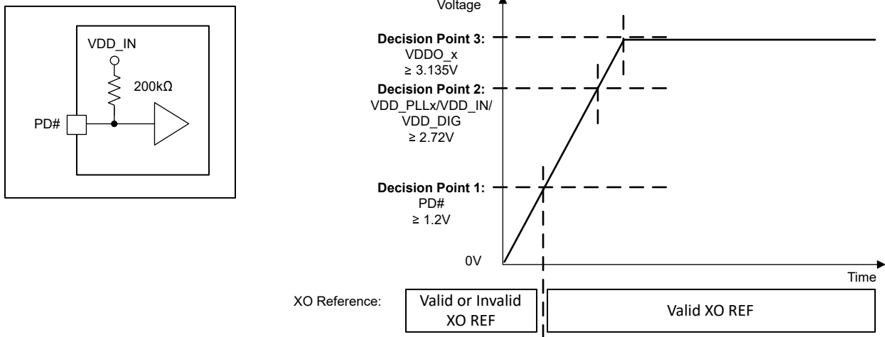
图 8-1. 从单电源轨上电的建议
