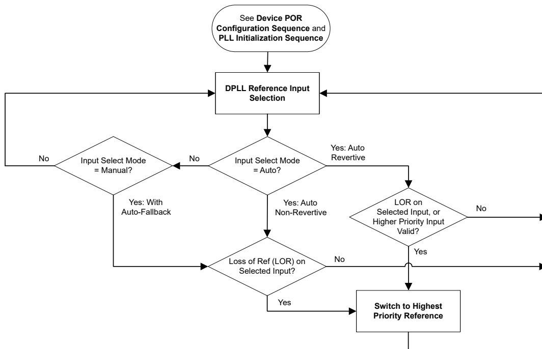
图 7-16. DPLL 基准输入选择流程图
