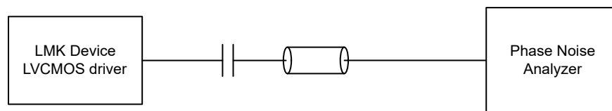
图 6-4. LVCMOS 输出相域测试配置
