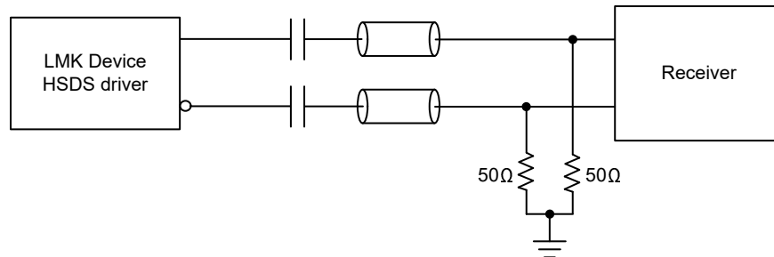
图 7-29. 交流耦合 HSDS 输出端接方法 2
