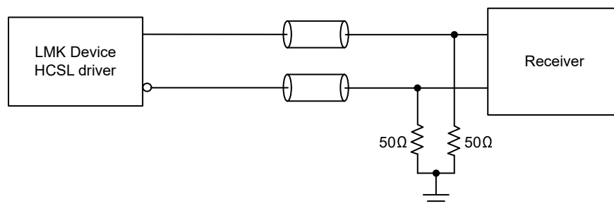
图 7-30. 直流耦合 HCSL 输出端接
