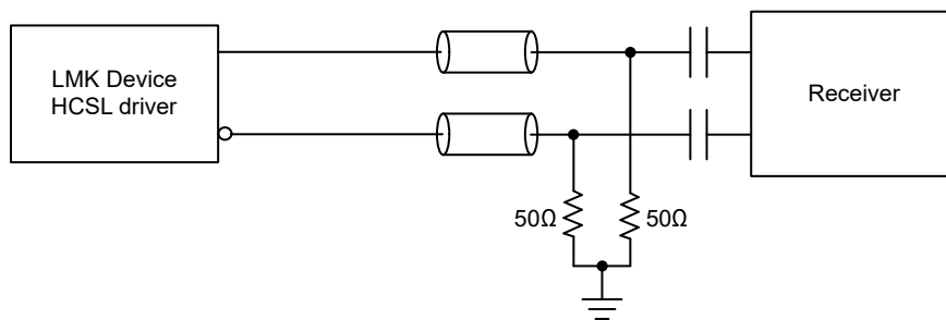
图 7-31. 交流耦合 HCSL 输出端接
