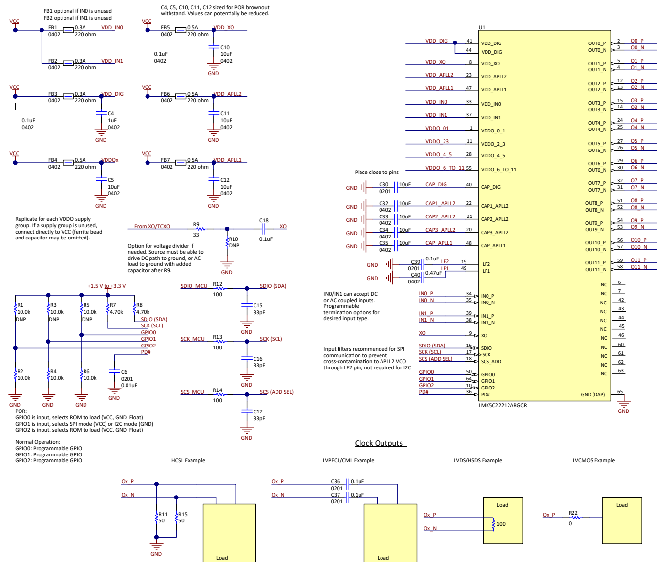
图 8-3. 参考原理图示例
