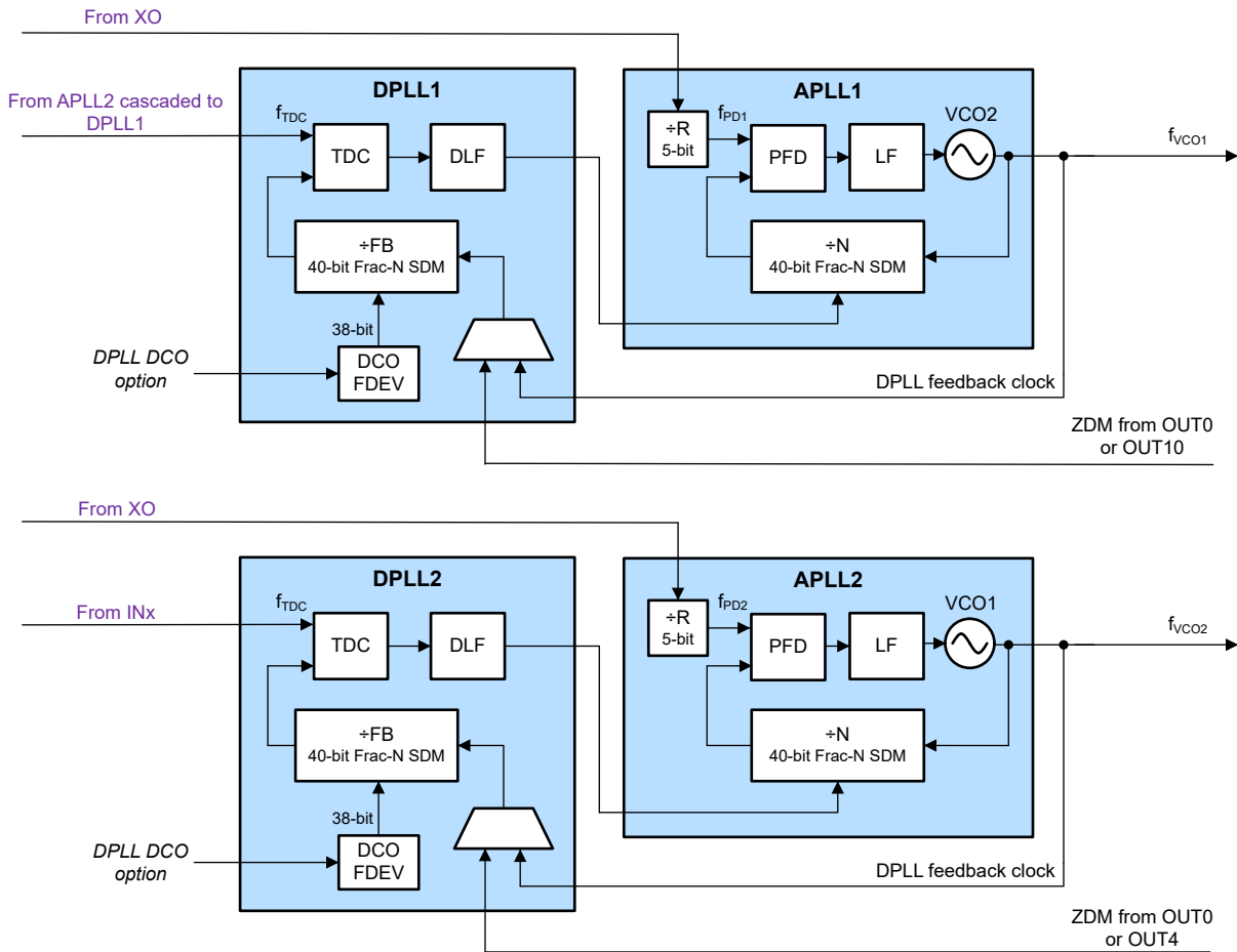
图 7-4. DPLL 级联模式
