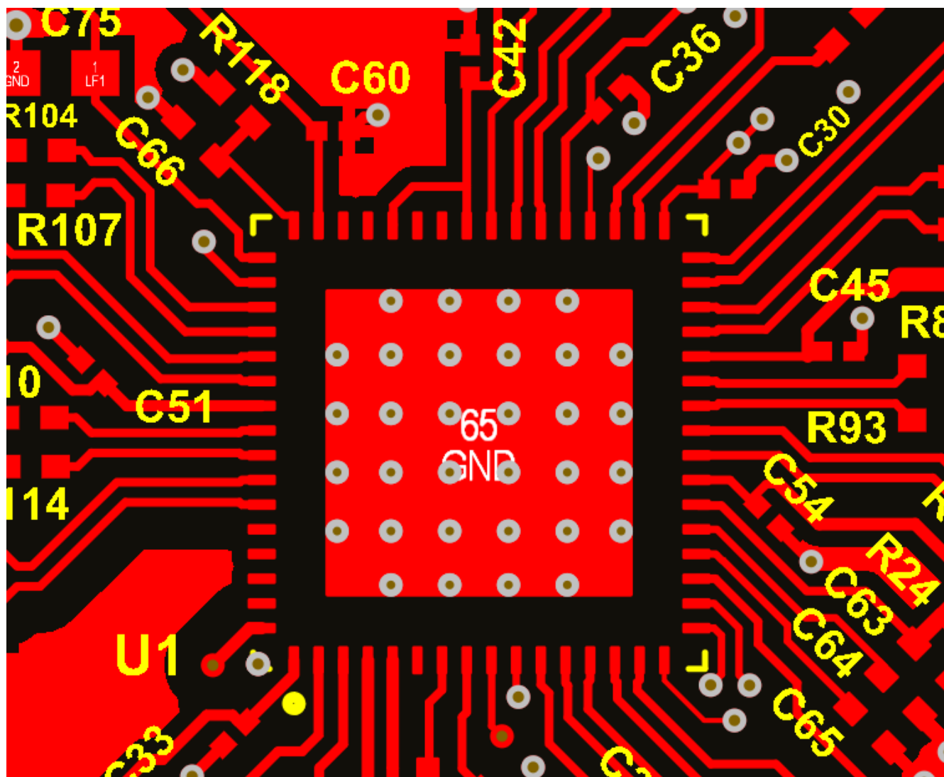
图 8-5. LMK5C22212A 的 PCB 布局示例，顶层
