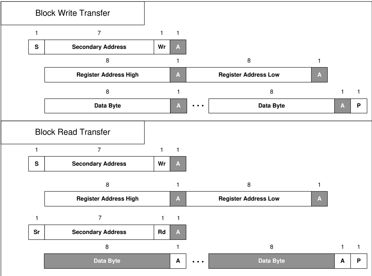
图 7-46. I 2 C 块寄存器传输
