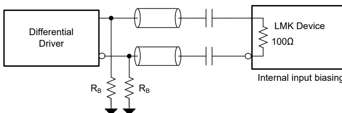
图 7-15. 交流耦合差分至基准 (INx)
