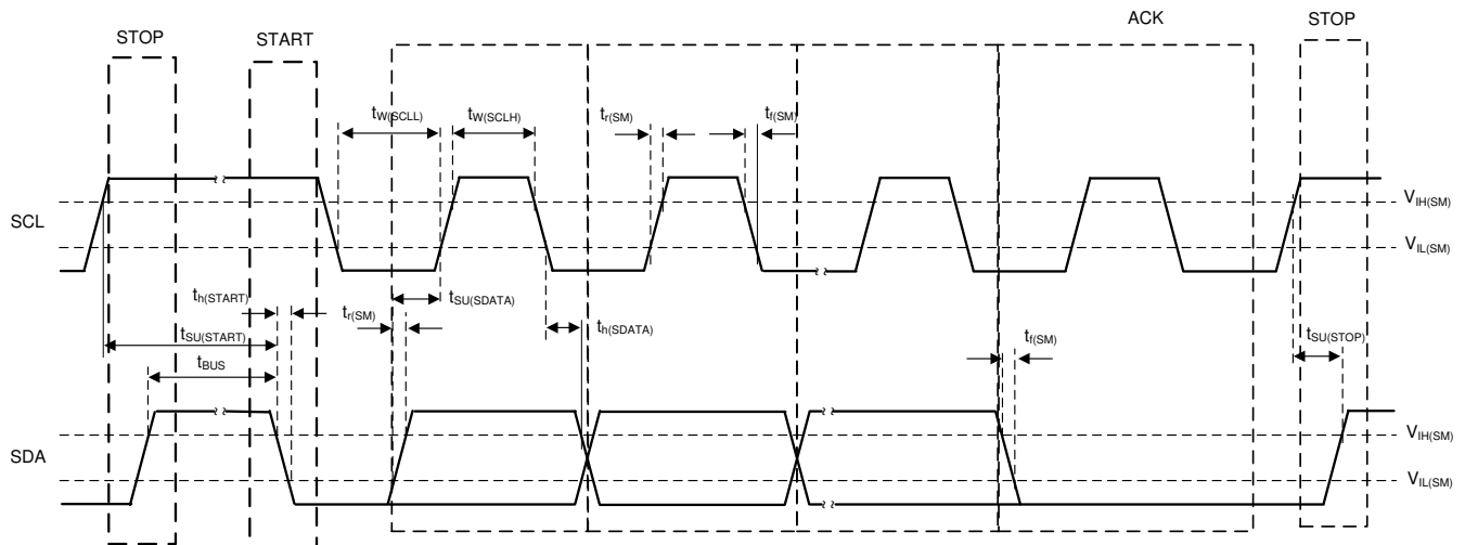
图 5-4. I²C 时序图
