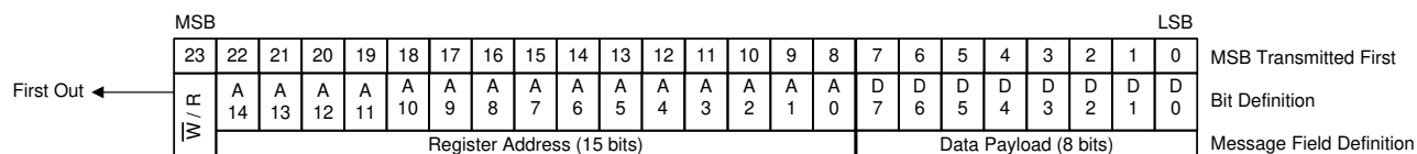
图 7-44. SPI 消息格式
