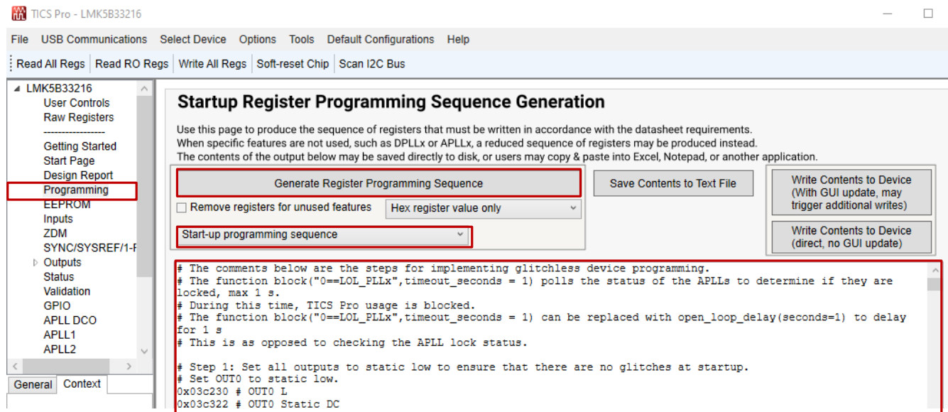
图 7-47. LMK5xxxxxx TICS Pro 编程页面 (v1.7.7.4 的屏幕截图。)
