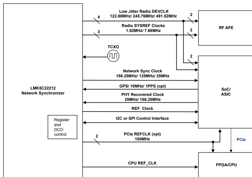
LMK5C22212A 典型系统方框图
