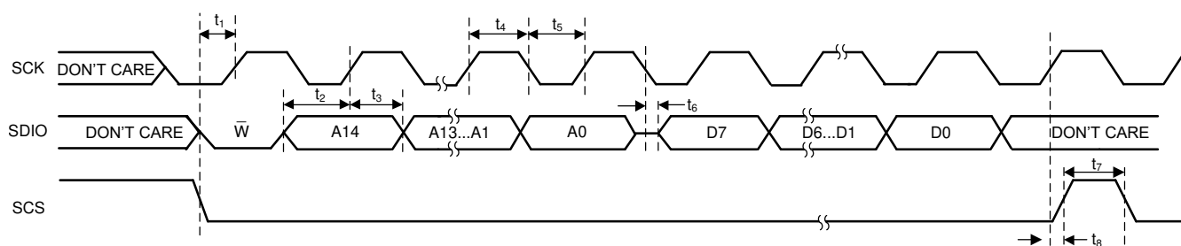
图 5-3. SPI 三线制读取时序图
