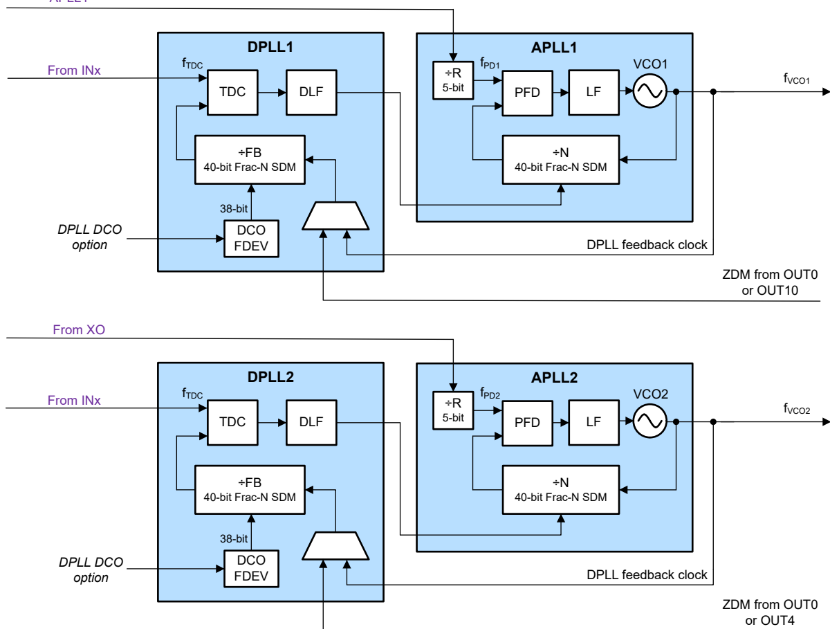
图 7-5. 启用 DPLL 的 APLL 级联示例
