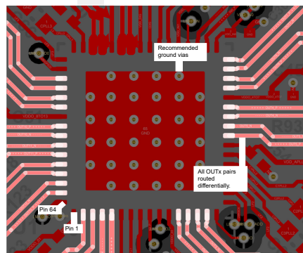
图 9-5. LMK5B33414 的 PCB 布局示例，顶层
