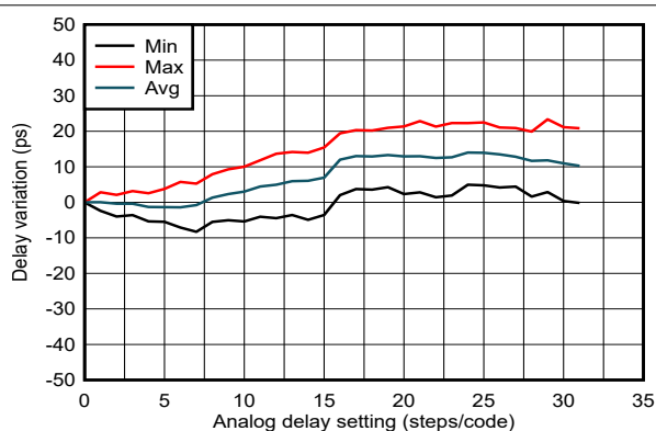
图 6-23. SYSREF/1PPS 延迟线性度与模拟延迟代码 4
