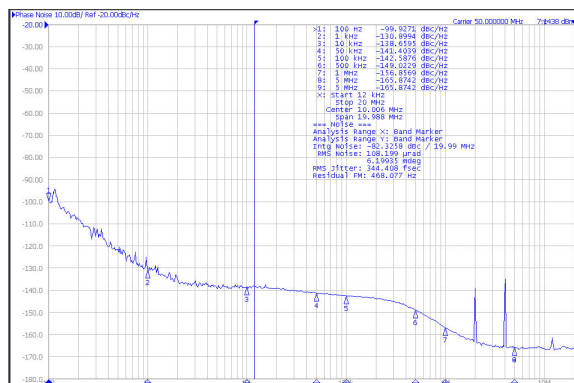
图 6-20. APLL1 的 50MHz HSDS 输出
