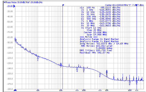
图 6-15. APLL2 的 161.1328125MHz HSDS 输出
