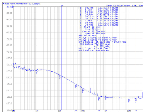
图 6-8. BAW APLL 的 312.5MHz HSDDS 输出
