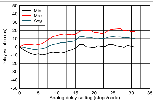
图 6-24. SYSREF/1PPS 延迟线性度与模拟延迟代码 5
