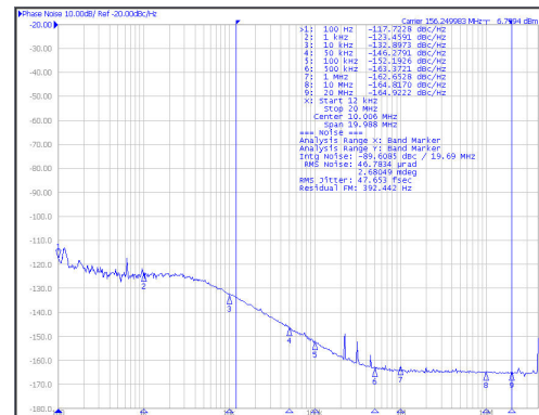
图 6-9. BAW APLL 的 156.25MHz HSDDS 输出
