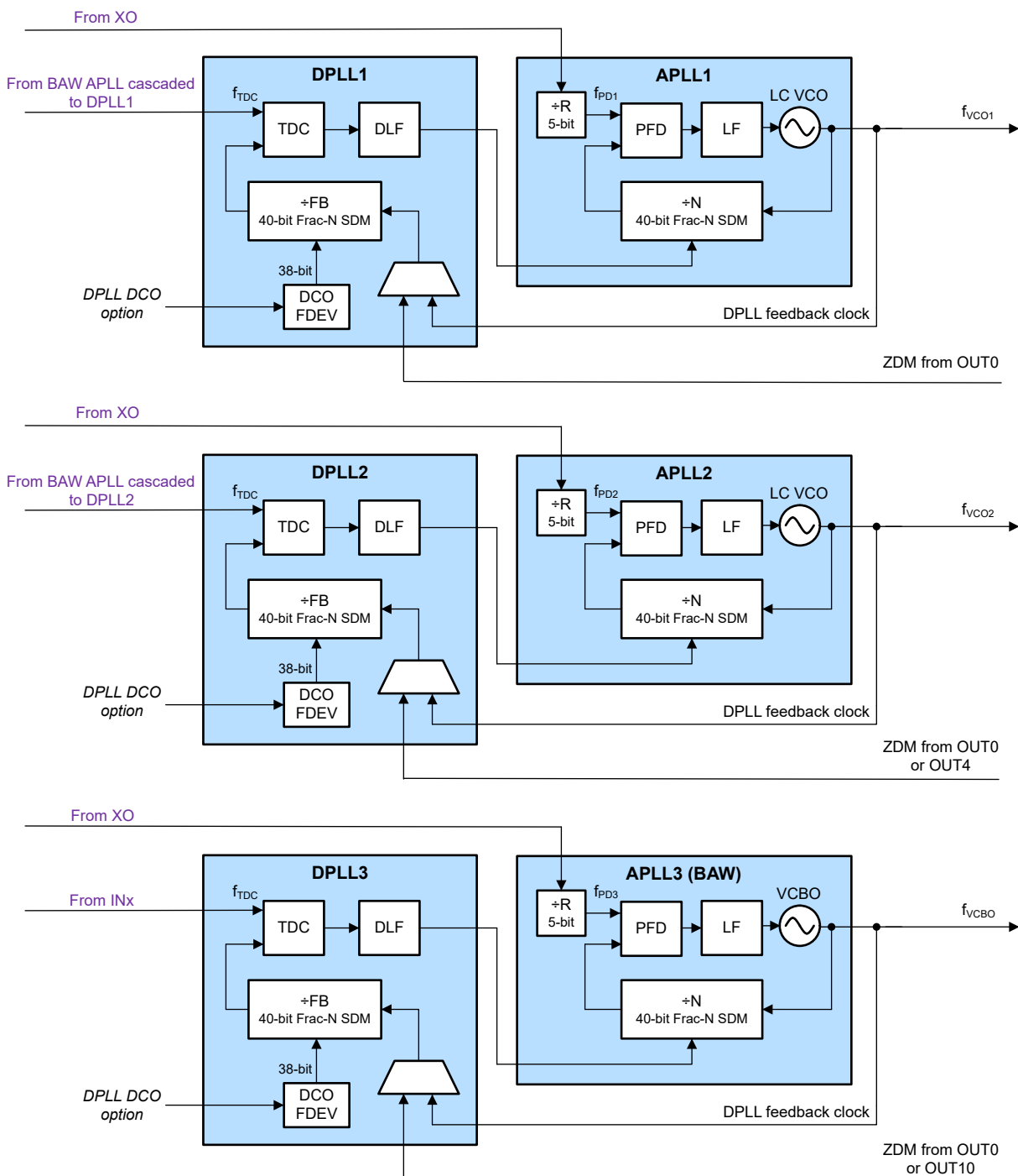
图 8-4. DPLL 级联模式
