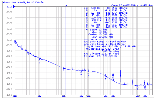
图 6-14. APLL2 的 212.5MHz HSDS 输出
