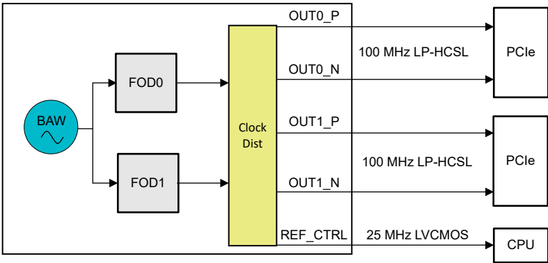
图 9-1. PCIe 应用
