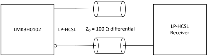
图 7-8. 将 LMK3H0102 LVCMOS 输出与 LP-HCSL 接收器相连接
