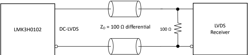
图 7-7. 将 LMK3H0102 LVCMOS 输出与直流 LVDS 接收器相连接
