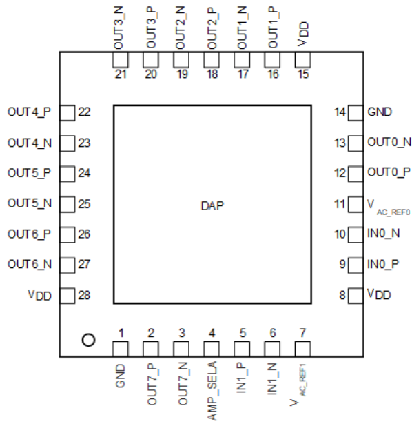
图 5-2. LMK1D2104L : RHD 封装 28 引脚 VQFN 顶视图
