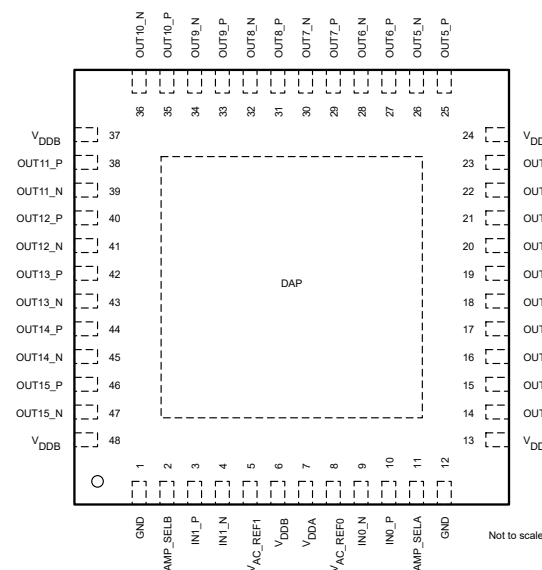
图 5-4. LMK1D2108L : RGZ 封装 48 引脚 VQFN 顶视图
