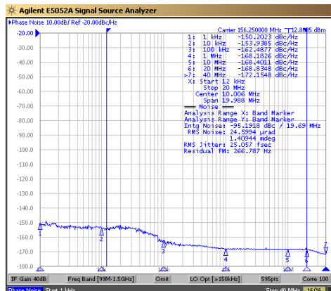
图 9-3. LMK1D210xL 参考相位噪声，156.25MHz， 25fs RMS ( 12kHz 至 20MHz )
