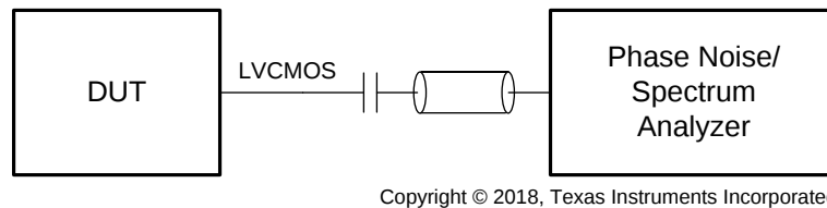
图 16. LVCMOS Output Phase Noise Test Configuration
