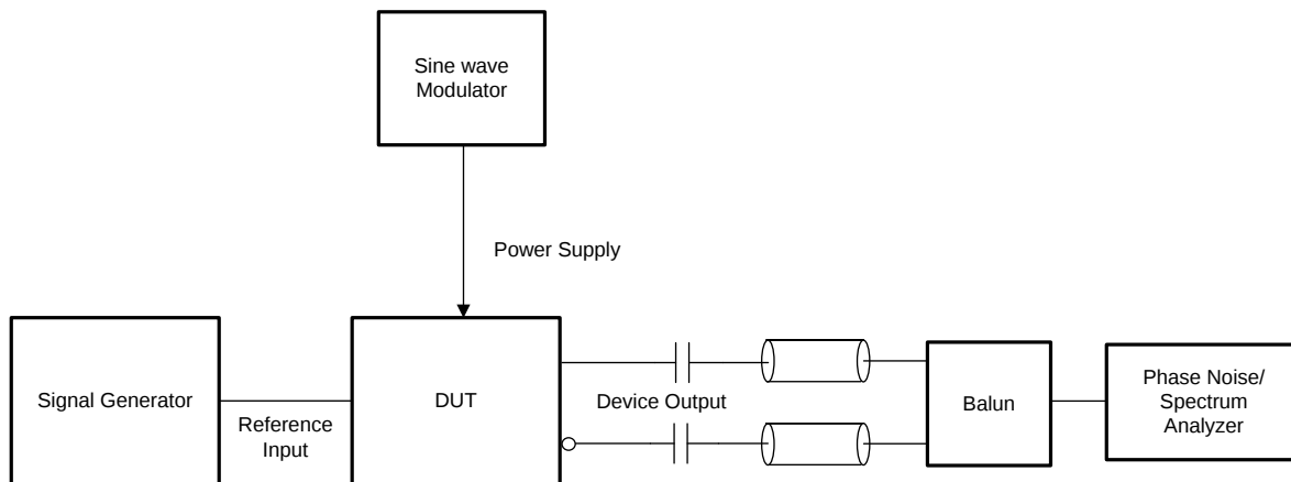
图 20. HCSL Output Phase Noise Test Configuration
