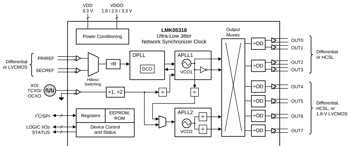
简化方框图
