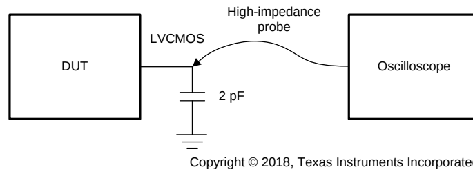
图 15. LVCMOS Output Test Configuration
