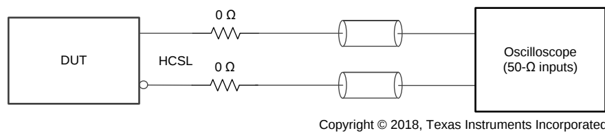
图 19. HCSL Output Test Configuration
