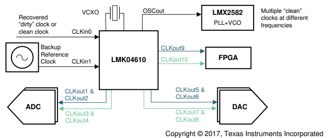
简化原理图
