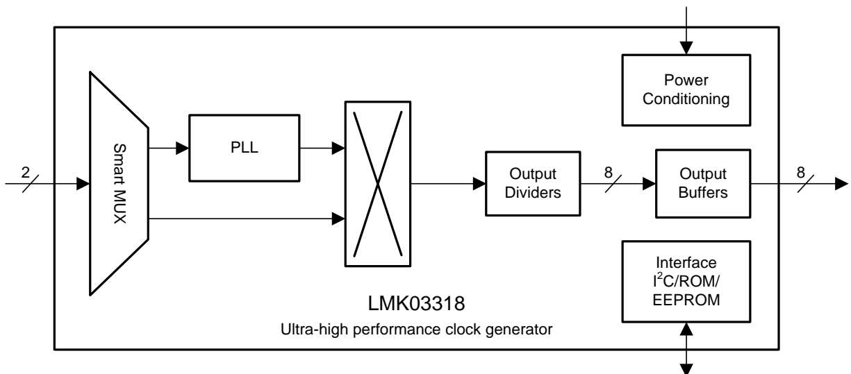
LMK03318 简化框图
