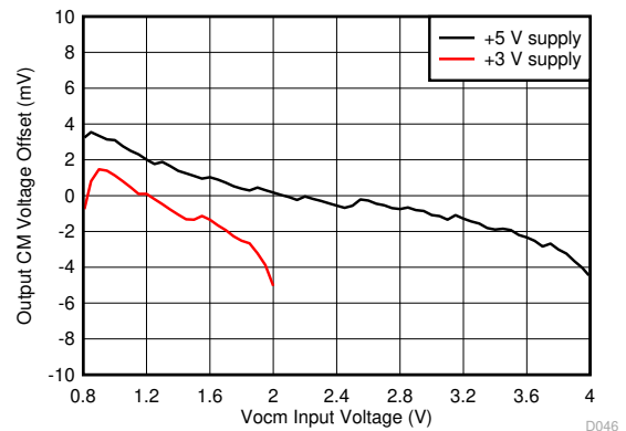
图 7-16. V_{\text{OCM}} Offset vs V_{\text{OCM}} Setting
