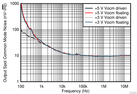
图 7-15. Output Common-Mode Noise
