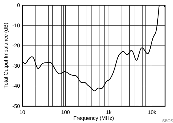
图 9. SE-DE Amplitude Imbalance
