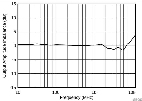
图 73. SE-DE Amplitude Imbalance
