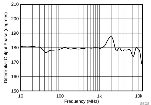
图 74. SE-DE Phase Imbalance
