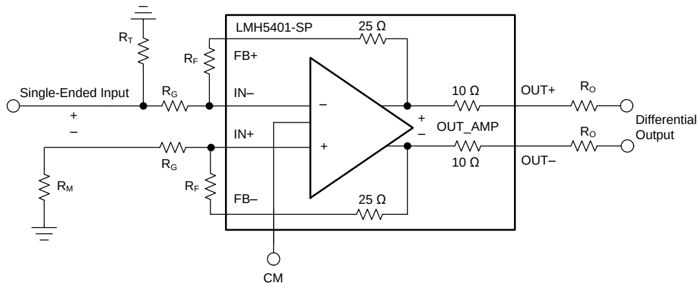
图 72. Active Balun
