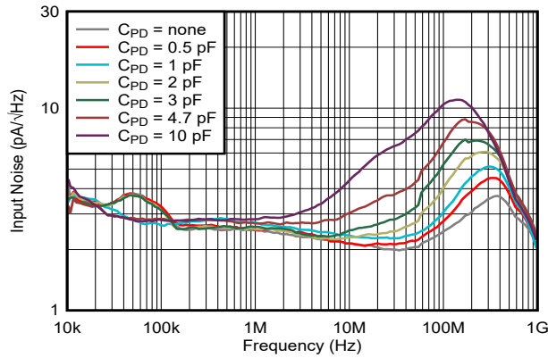
图 6-7. Input Noise Density vs Input Capacitance
