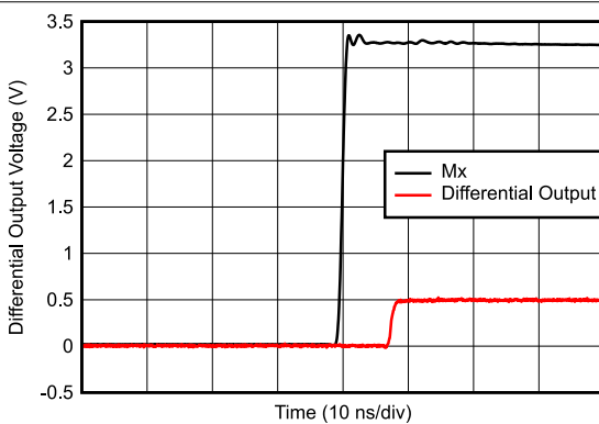
图 6-15. Turn-On Time
