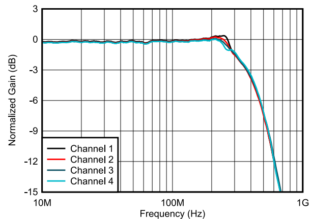
闭环带宽
