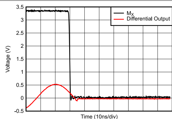
图 6-16. Turn-Off Time
