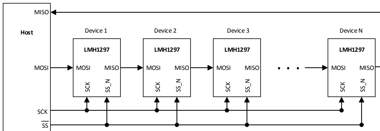
图 8-11. Daisy-Chain Configuration
