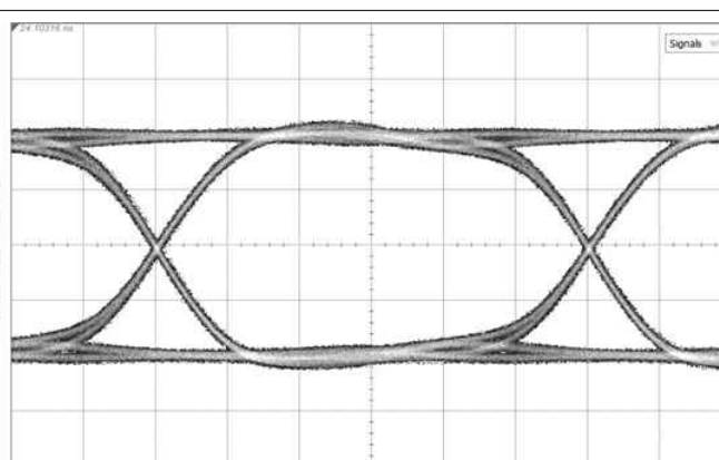
图 9-6. 11.88 Gbps, TL = 20" FR4, Reclocked
