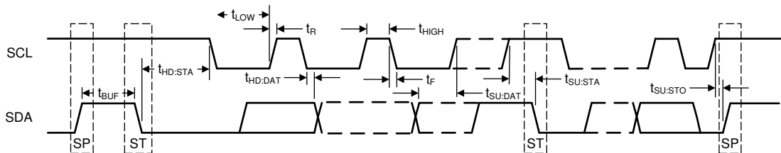
图 7-1. SMBus Timing Parameters
