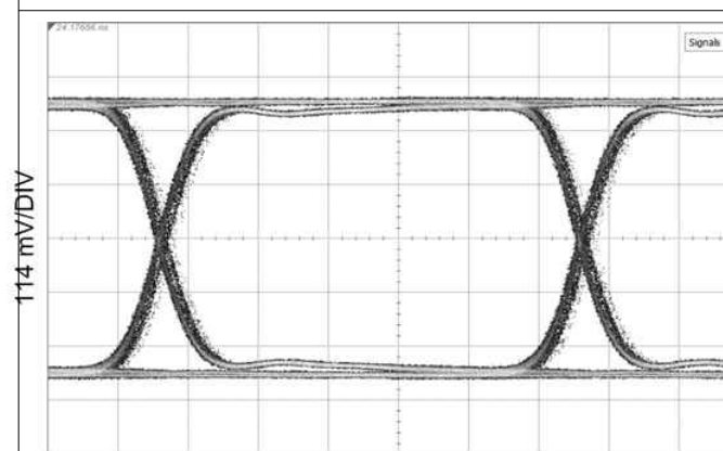
图 9-7. 5.94 Gbps, CC = 120-m Belden 1694A, Reclocked
