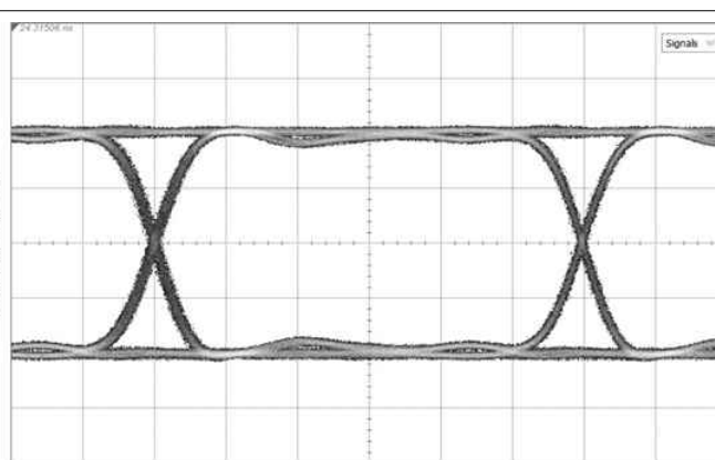
图 9-8. 5.94 Gbps, TL = 20" FR4, Reclocked
