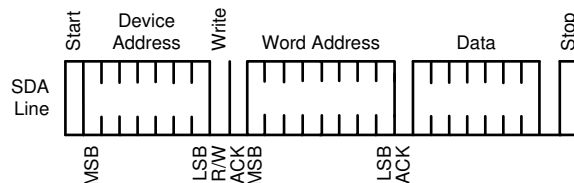
图 8-6. SMBus Write Operation
