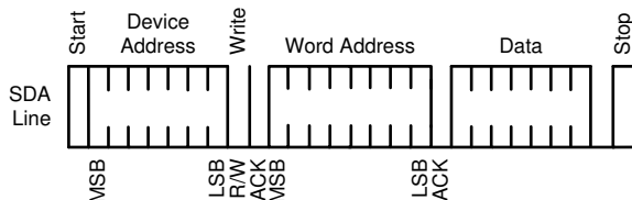
图 6-5. SMBus 写操作
