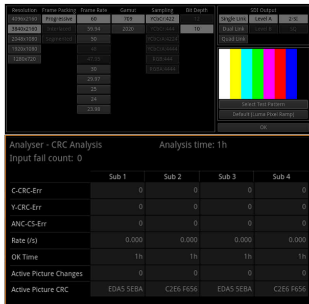
图 7-18. OUT0± BER 为 11.88Gbps (12G-SDI) , CC = 100m Belden 1694A , 经过时钟恢复
