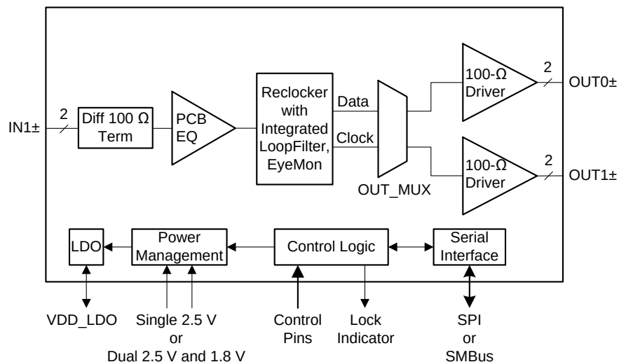
简化框图
