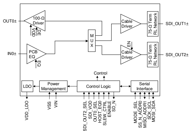
简化方框图
