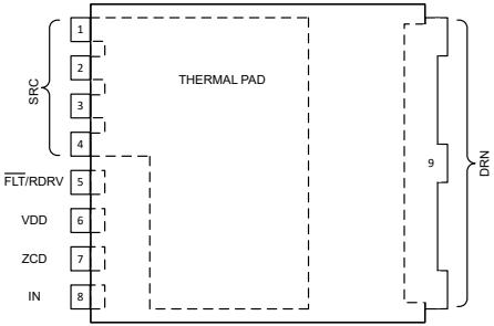
图 5-4. LMG3657R070 , TOLL 封装 (顶视图)
