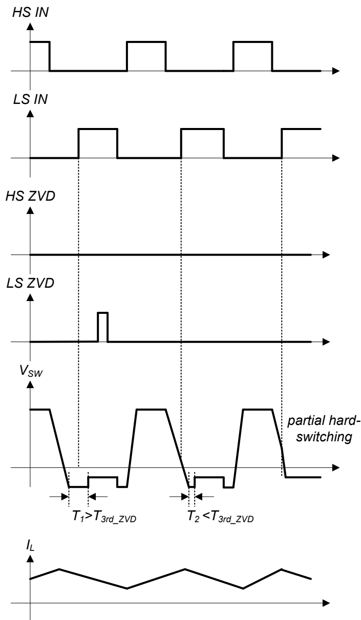
图 8-5. CCM 降压转换器中的 ZVD 功能
