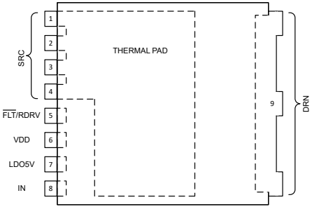
图 5-2. LMG3651R070 , TOLL 封装 (顶视图)
