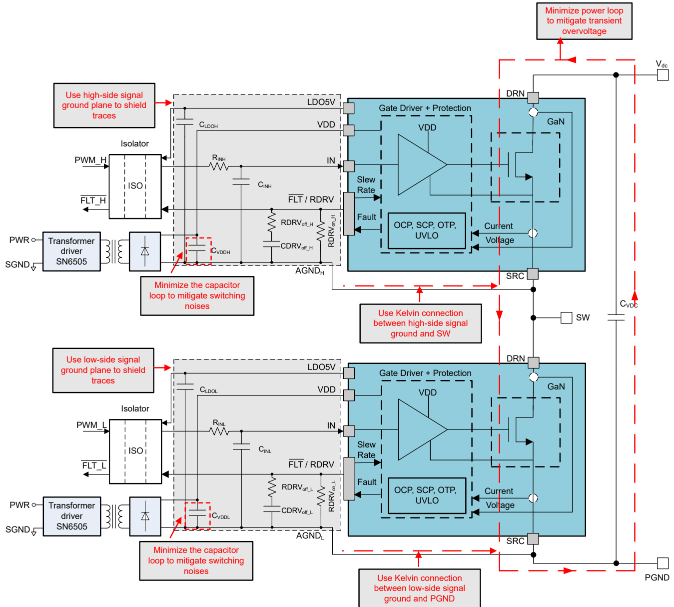
图 9-10. LMG3651R070 典型原理图及布局注意事项
