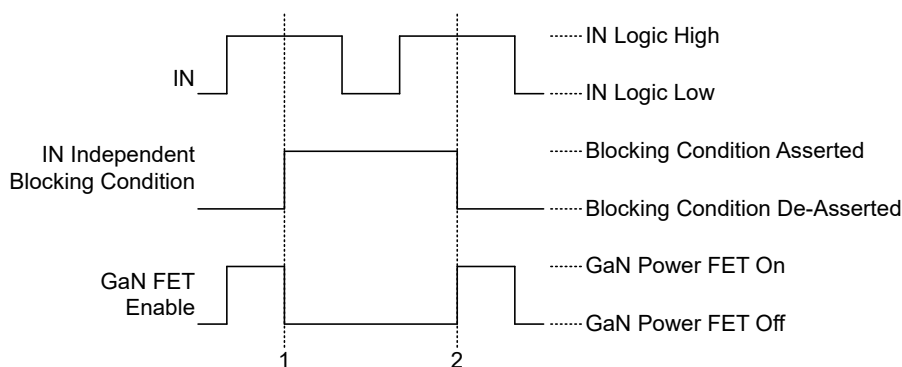
图 7-3. IN 独立阻断条件运行
