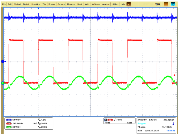
图 8-2. V_{IN} = 400VDC
