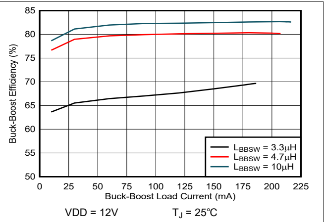
图 8-4. 当 I_{\text{BBSW,PK}} = I_{\text{BBSW,PK(high)}} 时降压/升压效率与负载之间的关系
