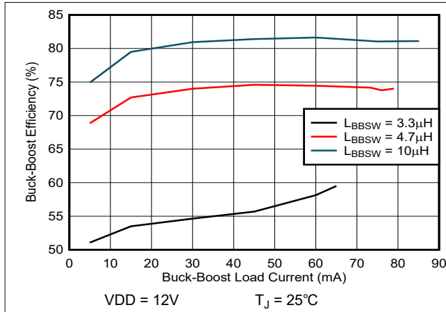
图 8-3. 当 I_{\text{BBSW,PK}} = I_{\text{BBSW,PK(low)}} 时降压/升压效率与负载之间的关系
