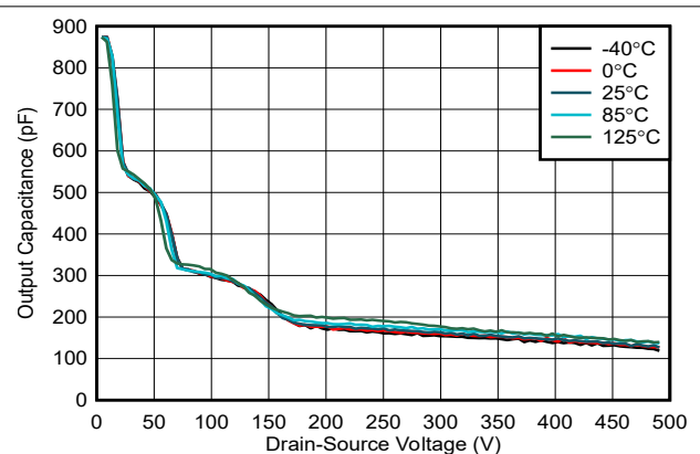
图 5-8. 输出电容与漏源电压之间的关系
