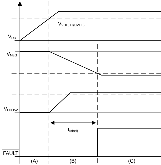
图 7-10. 启动时序图
