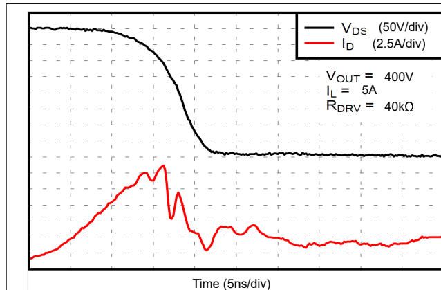
图 8-5. 应用示例中的导通波形
