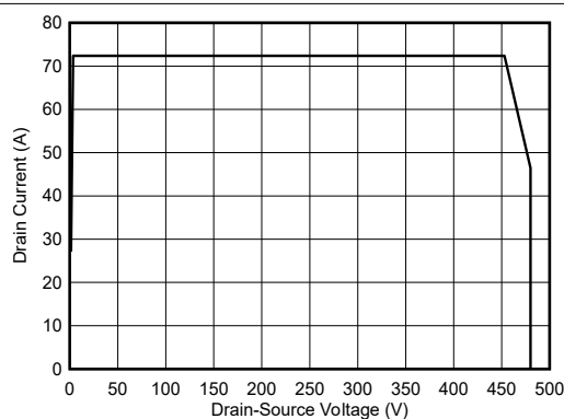
图 5-12. 最大安全工作区
