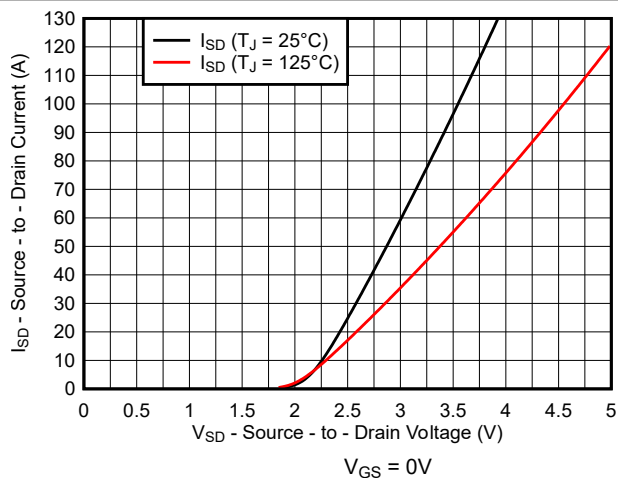
图 5-13. LMG3100R044 反向漏源特性
