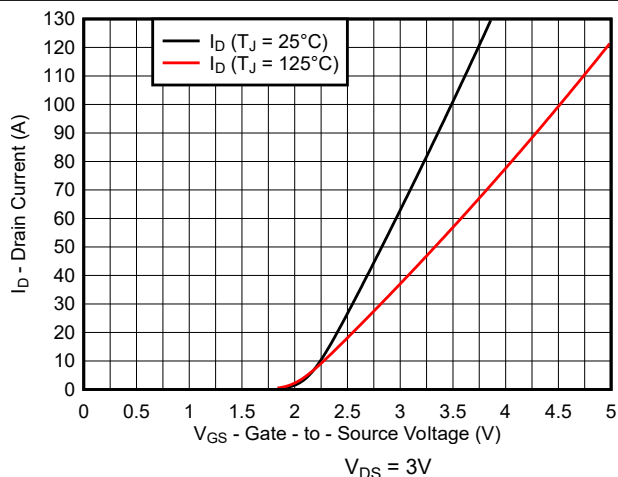
图 5-10. LMG3100R044 典型传输特性
