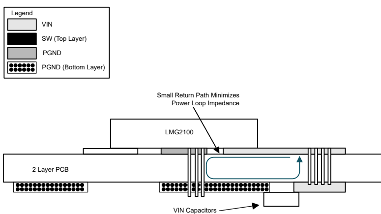
图 8-10. 具有返回路径的双层电路板横截面
