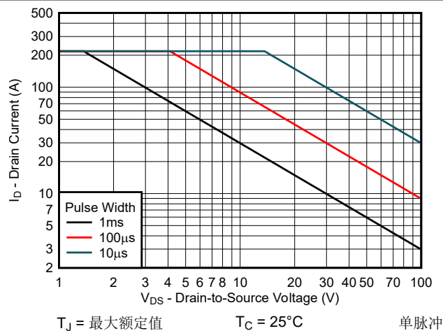
图 5-8. 安全工作区
