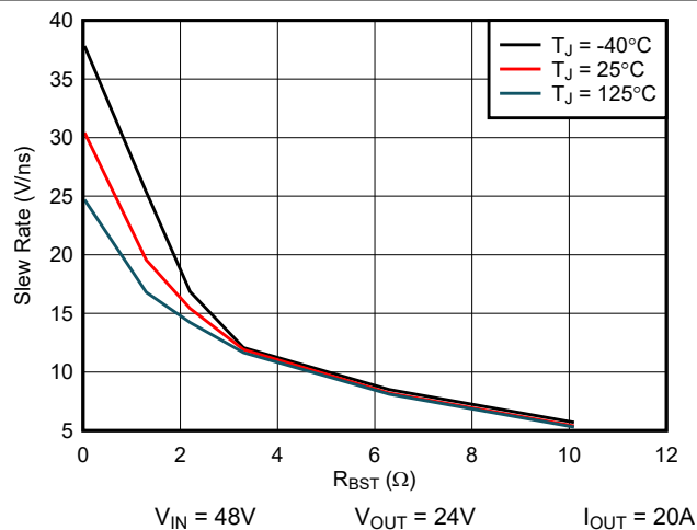
图 5-7. 针对使用 R_{BST} 的降压转换器的压摆率控制
