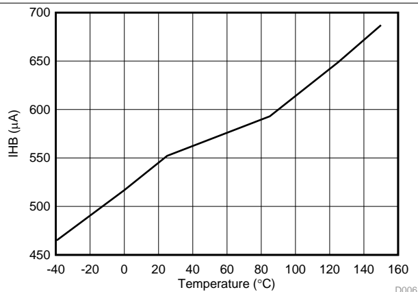
图 6. IHB vs Temperature
