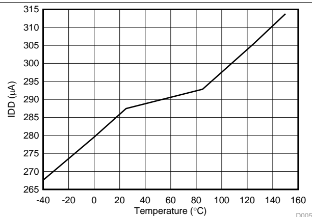
图 5. IDD vs Temperature
