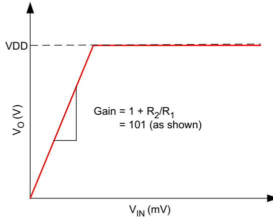
图 7-4. 输出响应
