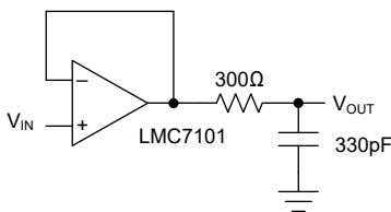
图 7-1. 330pF 容性负载的电阻式隔离
