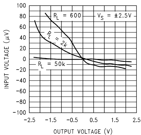
图 5-14. 输入电压与输出电压间的关系
