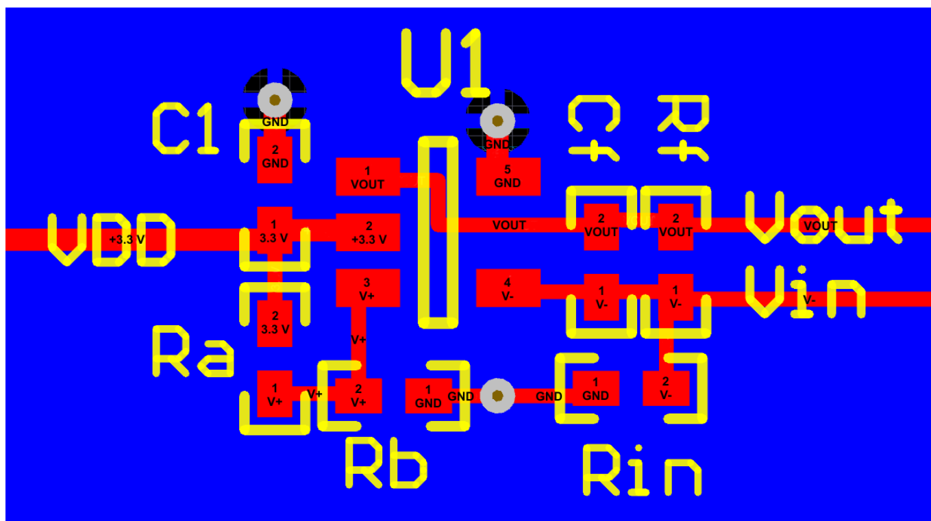
图 7-5. LMC7101 示例布局
