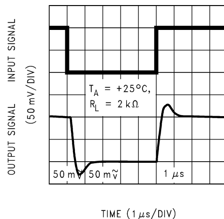
图 5-44. 反相大信号脉冲响应
