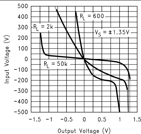
图 5-2. 输入电压与输出电压间的关系
