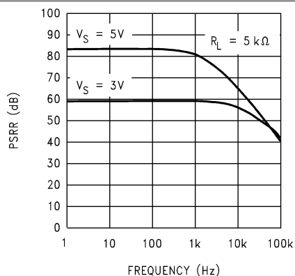
图 5-13. 正 PSRR 与频率间的关系
