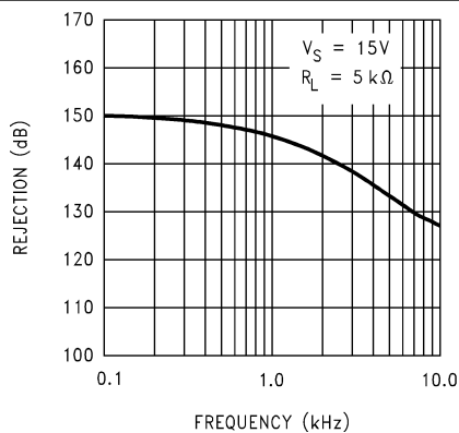
图 5-11. 串扰抑制与频率间的关系
