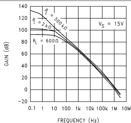
图 5-18. 开环频率响应
