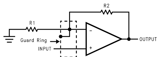
图 6-17. 同相放大器
