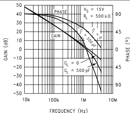
图 5-22. 增益和相位与容性负载间的关系
