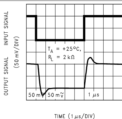
图 5-29. 同相小信号脉冲响应
