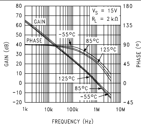
图 5-20. 开环频率响应与温度间的关系
