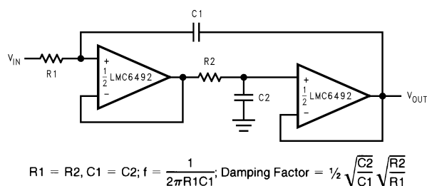
图 6-12. 轨到轨单电源低通滤波器
