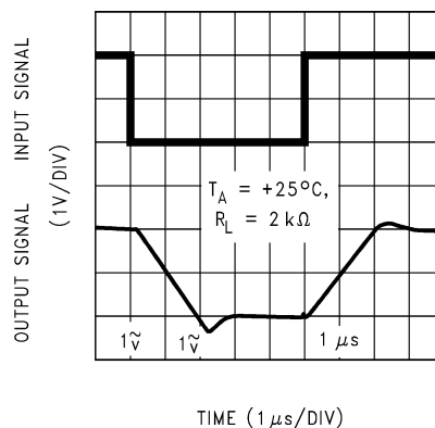
图 5-26. 同相大信号脉冲响应
