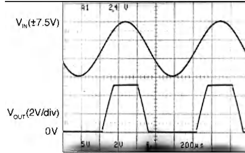
图 6-3. \pm 7.5V 的输入信号远远超过了图 6-3 中的 5V 电源，但由于 R_I 的原因，未产生相位反转
