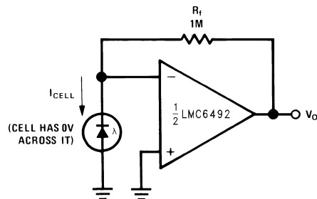
图 6-10. 光伏电池放大器
