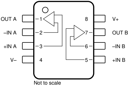
图 4-1. LMC6492 : D 封装 , 8 引脚 SOIC ( 顶视图 )
