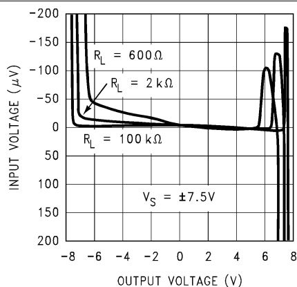
图 5-19. 输入电压与输出电压间的关系
