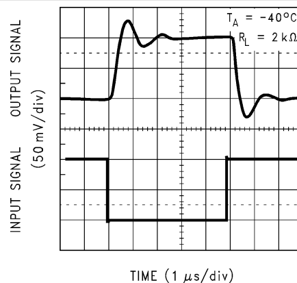
图 5-36. 反相小信号响应
