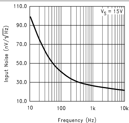
图 5-10. 输入噪声与频率间的关系
