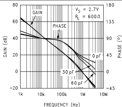
图 5-23. 增益和相位与容性负载间的关系
