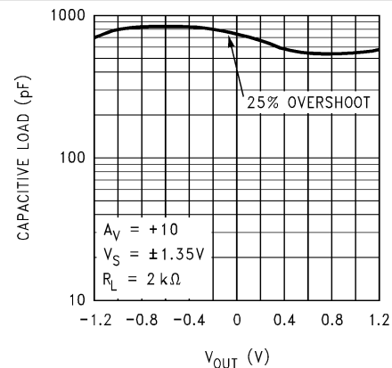
图 5-41. 稳定性与容性负载间的关系
