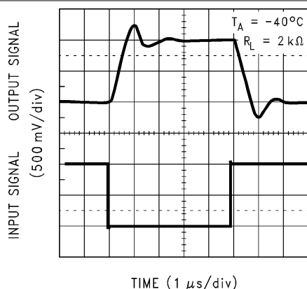
图 5-33. 反相大信号响应
