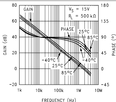
图 5-21. 频率响应与温度间的关系
