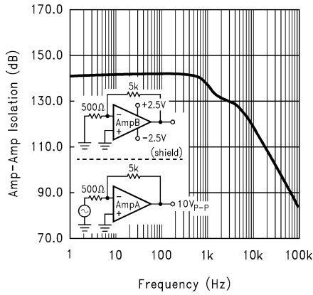
图 5-13. 放大器间隔离与频率间的关系
