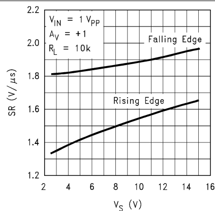
图 5-24. 压摆率与电源电压间的关系
