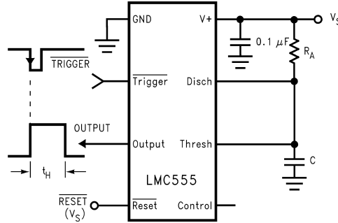
图 7-2. 单稳 (一次性)
