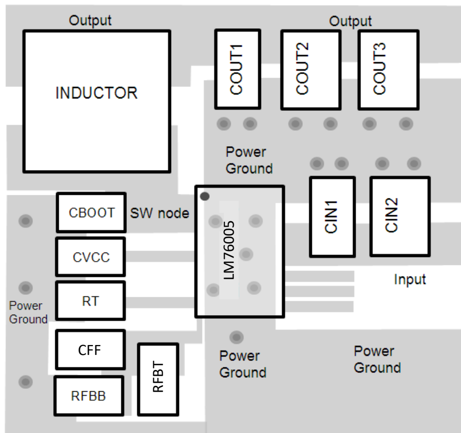
图 10-3. LM76005 Layout
