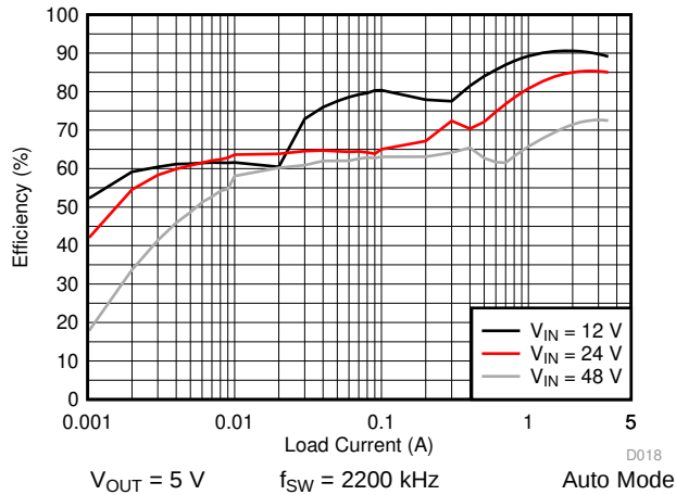
图 29. LM76003 Efficiency
