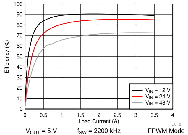
图 30. LM76003 Efficiency
