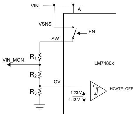
图 9-4. 编程过压阈值和电池检测
