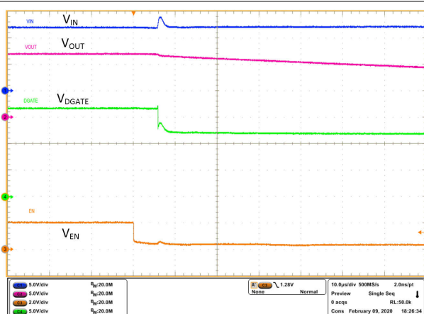
图 10-16. 关断延迟 - DGATE
