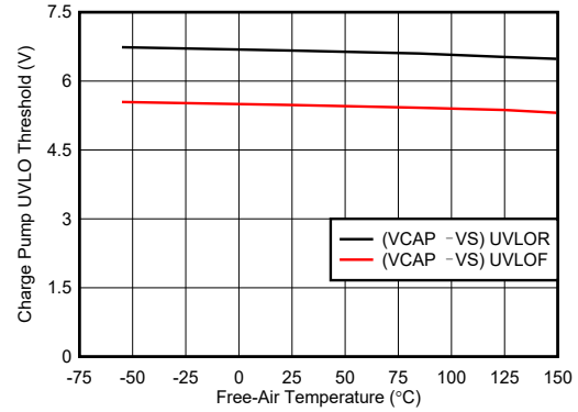
图 7-10. 电荷泵 UVLO 阈值与温度间的关系
