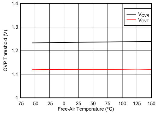
图 7-9. OVP 阈值与温度间的关系
