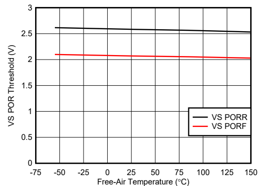
图 7-12. VS POR 阈值与温度间的关系
