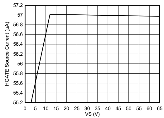
图 7-14. HGATE 电流 (IHGATE) 与电源电压间的关系
