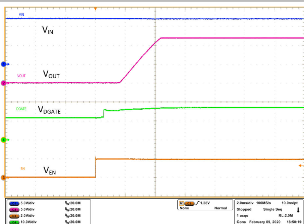
图 10-10. 通过使能使 DGATE 导通
