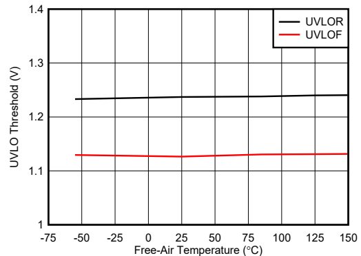
图 7-8. UVLO 阈值与温度间的关系
