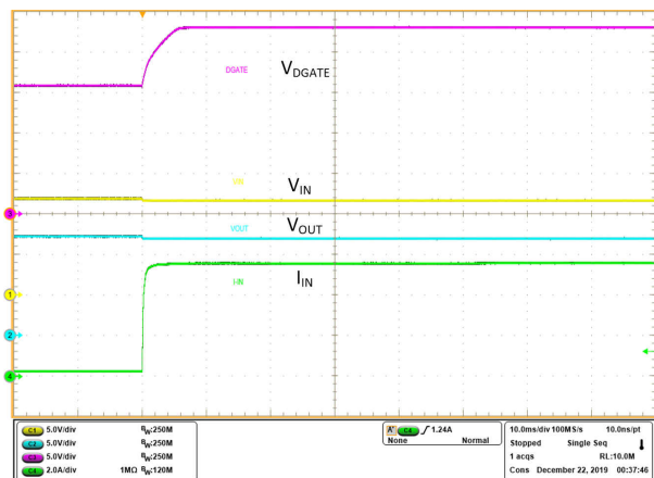
图 10-18. 负载瞬态，100mA 至 5A
