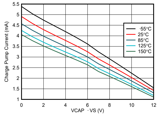
图 7-4. V_S \geq 12V 时的电荷泵 V-I 特性
