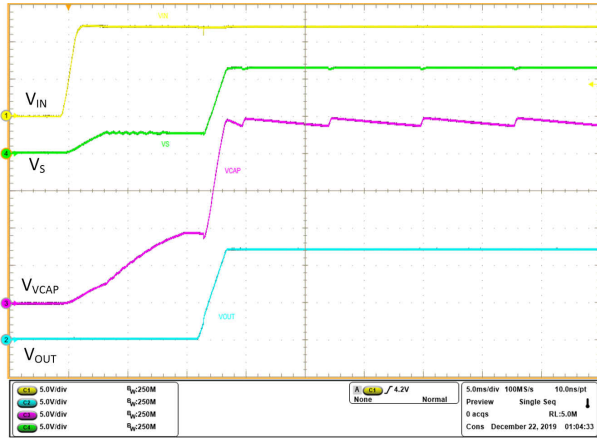
图 10-27. 上电 12V - 电荷泵 VCAP
