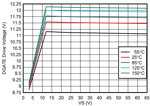
图 7-5. DGATE 驱动电压与电源电压间的关系
