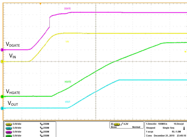
图 10-2. 启动电压为 12V，EN 拉至 VIN
