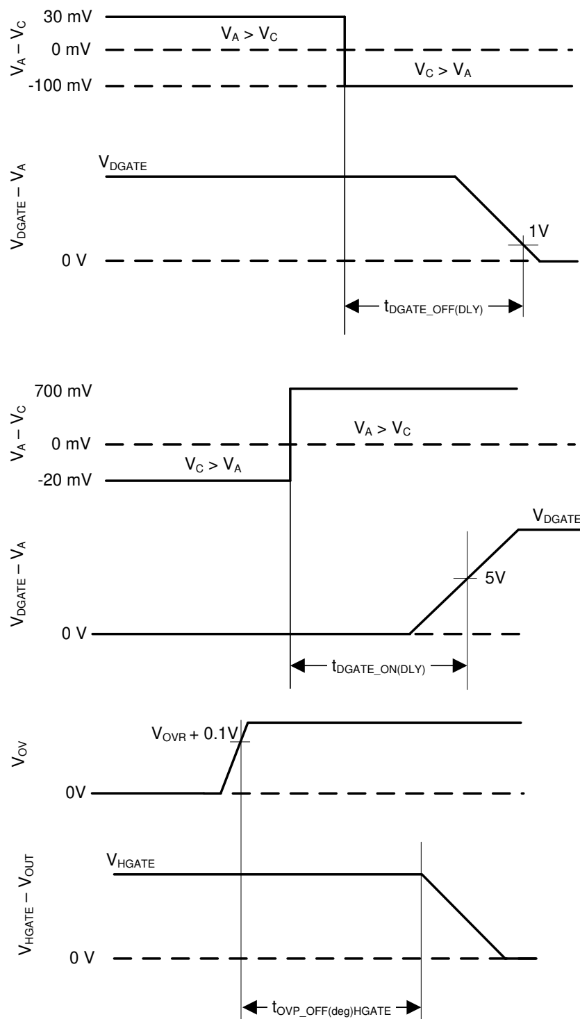
图 8-1. 时序波形
