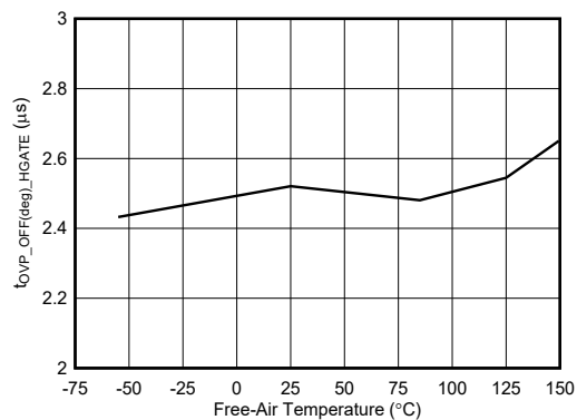
图 7-13. OV 期间的 HGATE 关断延迟
