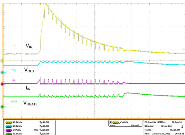
图 10-21. 未抑制的负载突降 200V - 输出钳位
