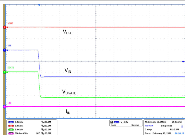
图 10-4. 反向输入电压为 -14V
