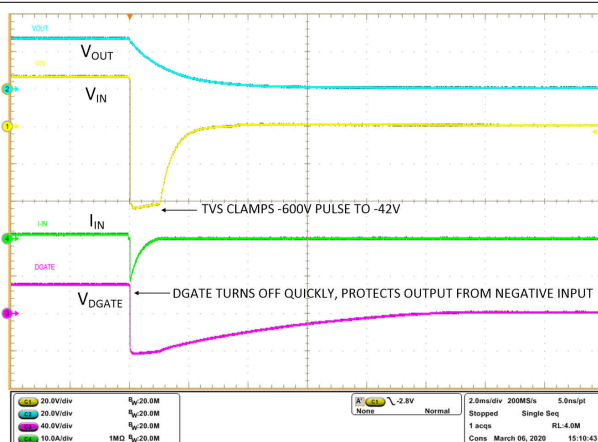
图 10-23. ISO 7637-2 脉冲 1 - 600V 50 \Omega
