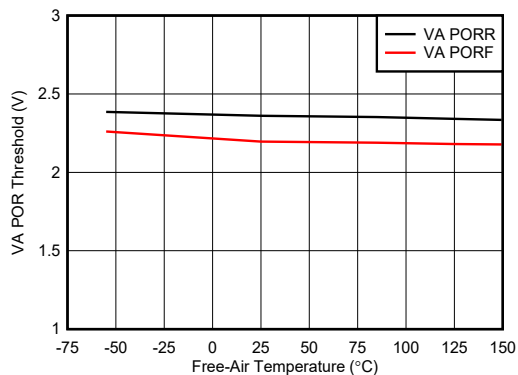
图 7-11. VA POR 阈值与温度间的关系
