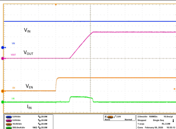
图 10-9. 通过使能使输出导通
