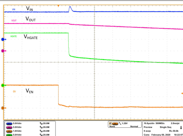
图 10-17. 关断延迟 - HGATE
