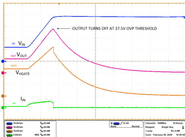
图 10-13. 过压保护
