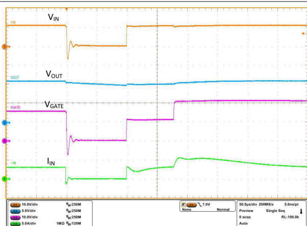
图 9-5. Input Micro-Short - LV124 E10 TC 2 100 \mu s
