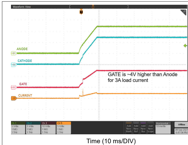
图 9-10. Startup With 3-A Load
