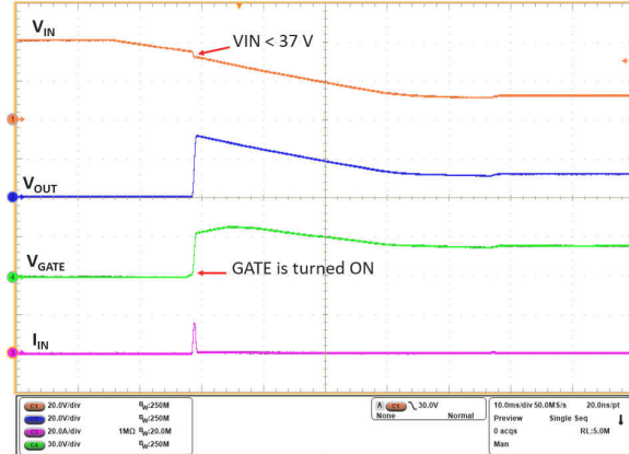
图 10-9. Overvoltage Recovery
