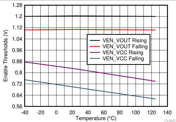
图 7-8. Enable Thresholds
