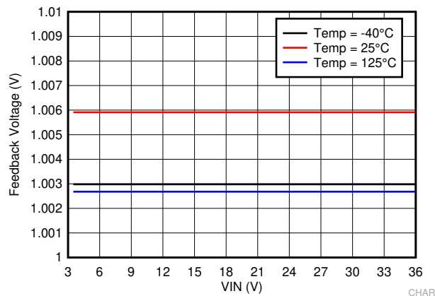
图 7-3. Feedback Voltage
