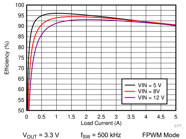
图 9-6. LM73605-Q1 Efficiency
