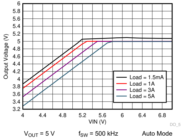
图 9-39. LM73605-Q1 Dropout Curve
