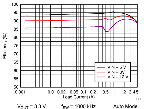
图 9-10. LM73605-Q1 Efficiency
