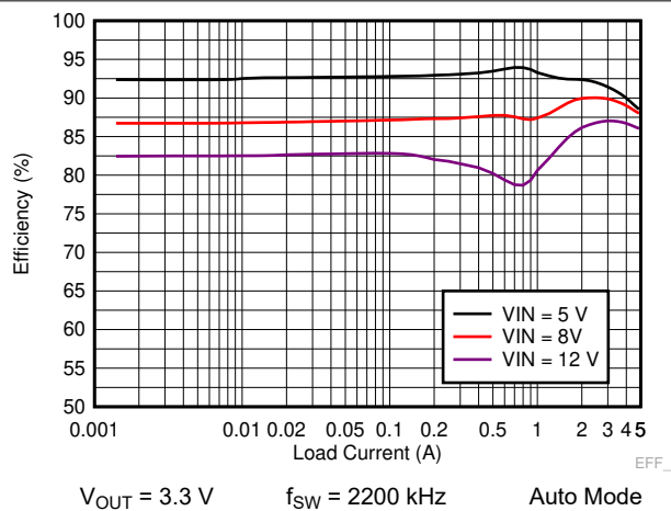
图 9-7. LM73605-Q1 Efficiency
