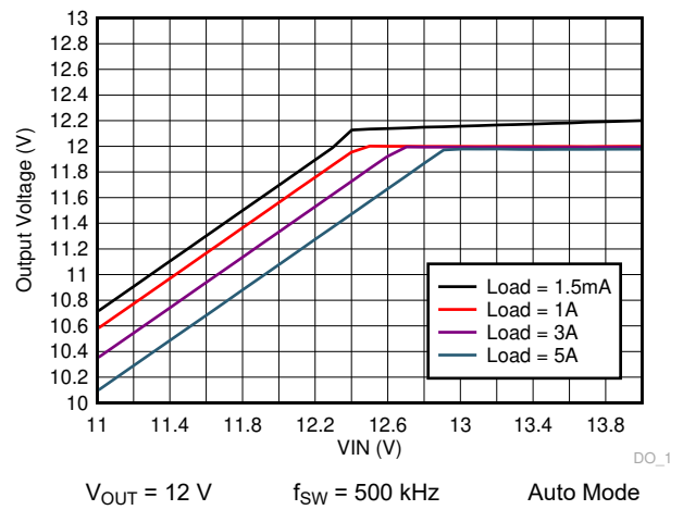
图 9-44. LM73605-Q1 Dropout Curve
