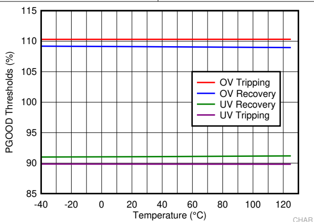
图 7-9. PGOOD Thresholds
