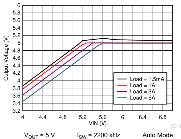
图 9-37. LM73605-Q1 Dropout Curve
