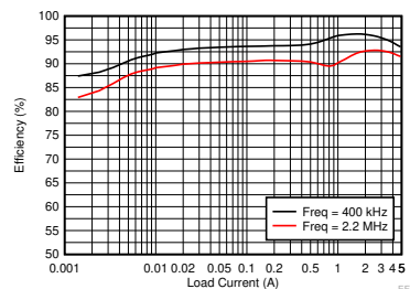
效率与负载电流 V_{OUT} = 5V , V_{IN} = 12V , 自动模式
