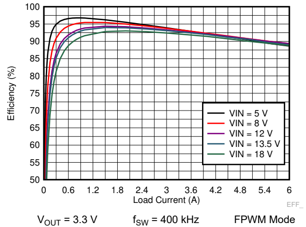
图 9-4. LM73606-Q1 Efficiency
