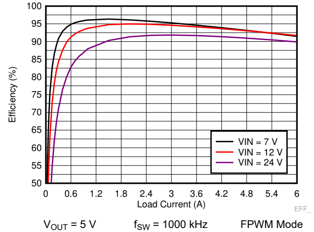
图 9-16. LM73606-Q1 Efficiency
