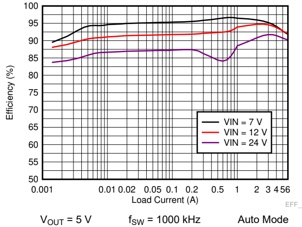
图 9-15. LM73606-Q1 Efficiency
