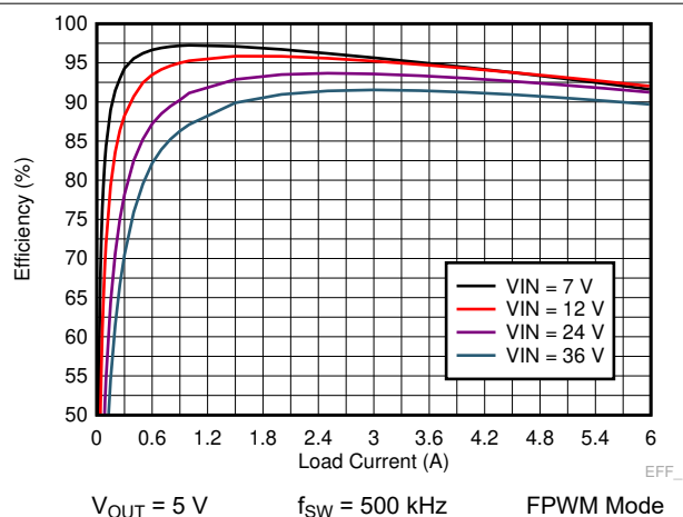
图 9-14. LM73606-Q1 Efficiency
