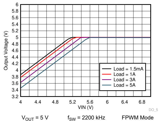
图 9-38. LM73605-Q1 Dropout Curve
