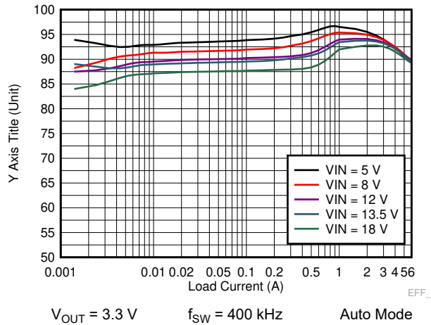
图 9-3. LM73606-Q1 Efficiency
