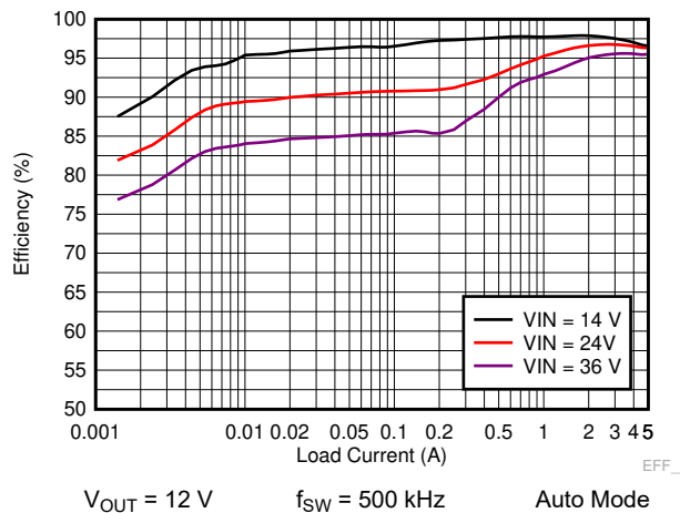
图 9-19. LM73605-Q1 Efficiency
