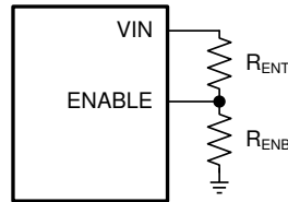
图 8-5. System UVLO
