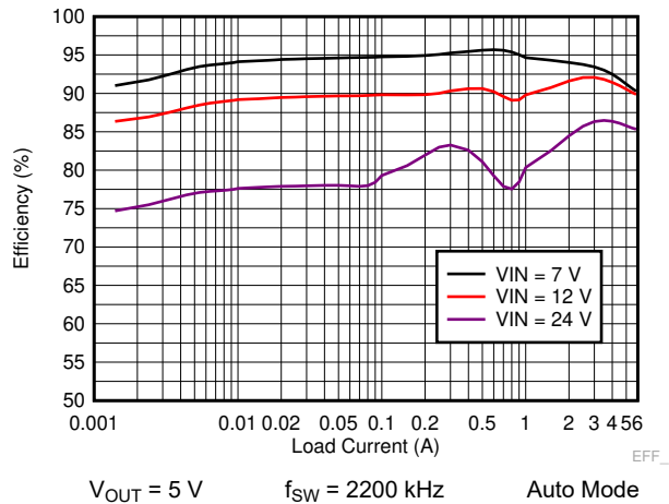
图 9-17. LM73606-Q1 Efficiency
