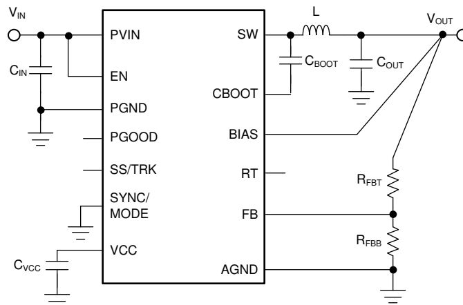
图 9-1. LM73605-Q1/6-Q1 Basic Schematic
