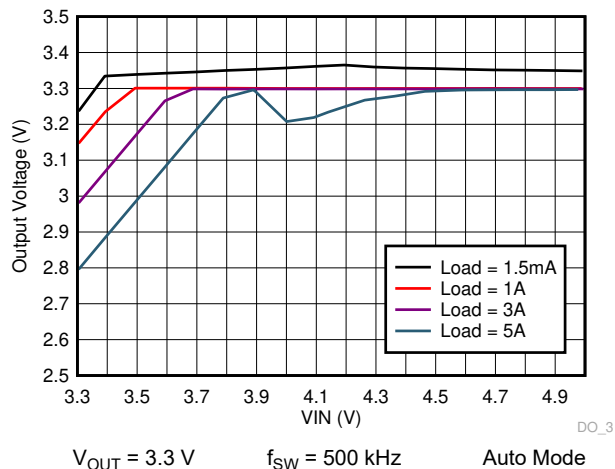
图 9-43. LM73605-Q1 Dropout Curve
