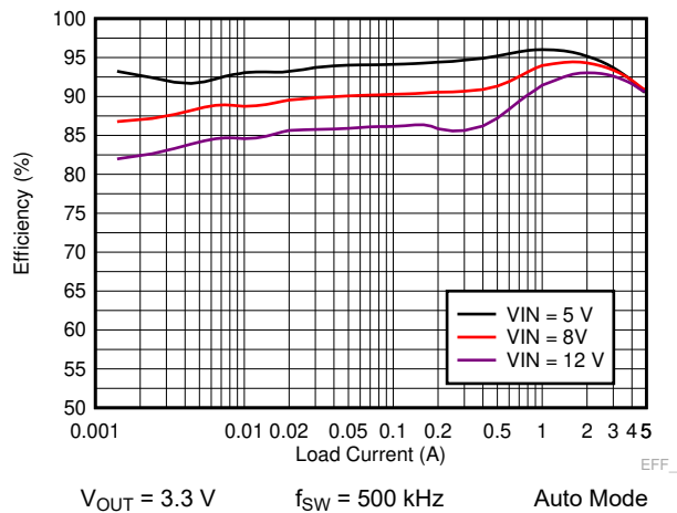
图 9-5. LM73605-Q1 Efficiency
