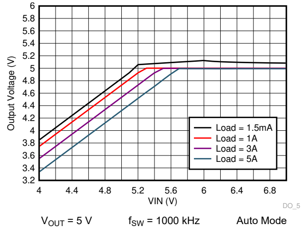
图 9-40. LM73605-Q1 Dropout Curve
