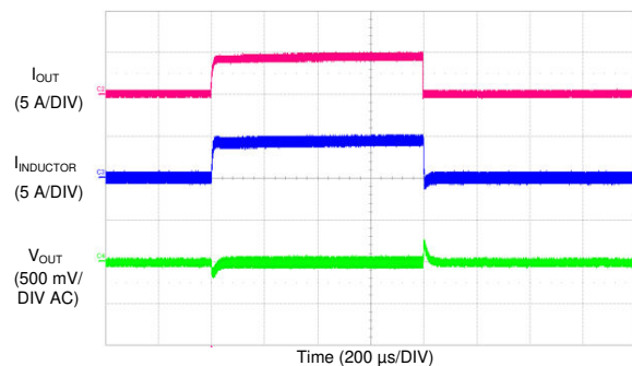
图 9-58. LM73606-Q1 Load Transients
