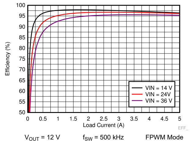
图 9-20. LM73605-Q1 Efficiency
