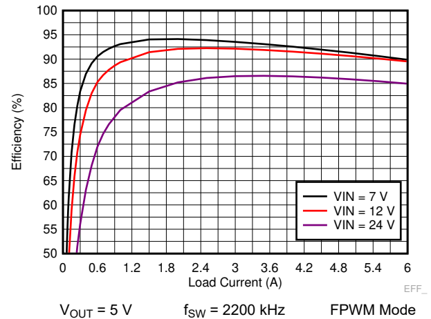
图 9-18. LM73606-Q1 Efficiency
