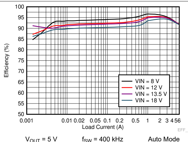
图 9-11. LM73606-Q1 Efficiency
