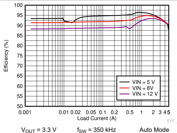
图 9-9. LM73605-Q1 Efficiency
