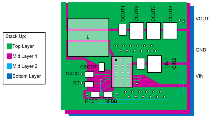
图 9-3. LM73605-Q1/6-Q1 Layout Example
