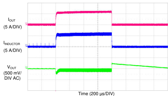
图 9-57. LM73606-Q1 Load Transients
