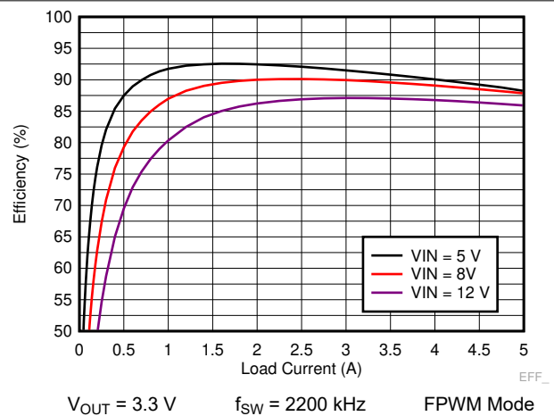
图 9-8. LM73605-Q1 Efficiency
