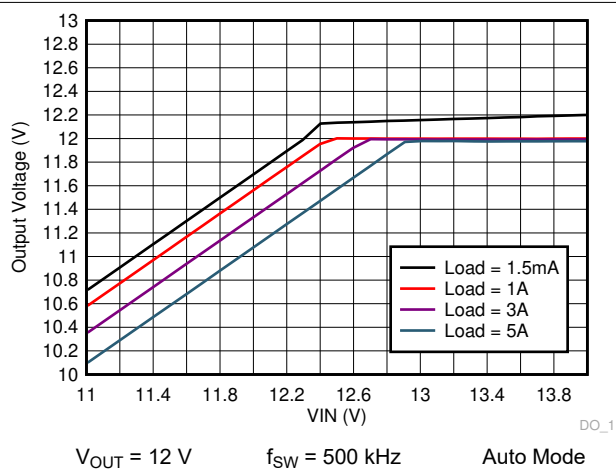
图 9-44. LM73605-Q1 Dropout Curve
