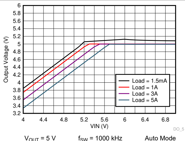
图 9-40. LM73605-Q1 Dropout Curve
