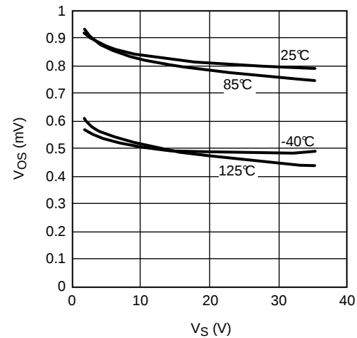
图 10. V_{OS} 与 V_S 间的关系 (单位 3)
