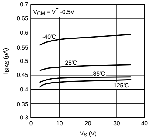
图 27. I_{\text{BIAS}} 与 V_{\text{S}} 间的关系
