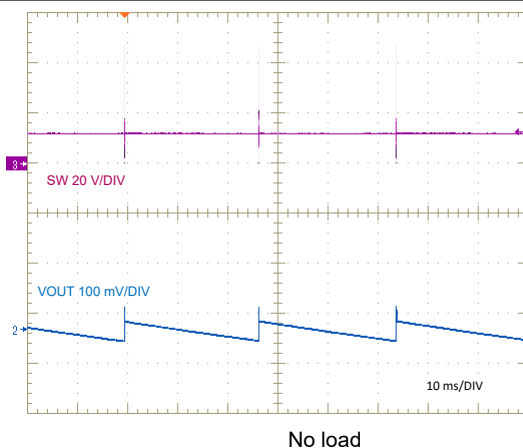
图 8-23. PFM Switching
