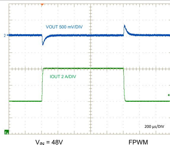
图 8-27. Load Transient, 4A to 8A
