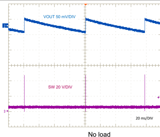
图 8-12. PFM Switching
