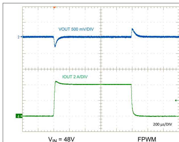
图 8-26. Load Transient, 0A to 4A
