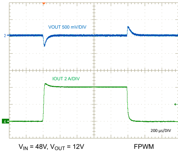
图 6-5. Load Transient, 0A to 4A
