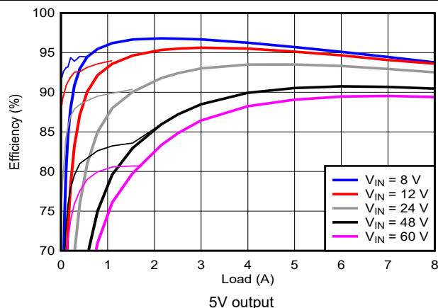
图 8-9. Efficiency versus I_{OUT}
