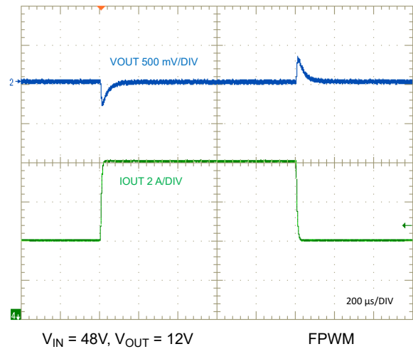
图 6-6. Load Transient, 4A to 8A
