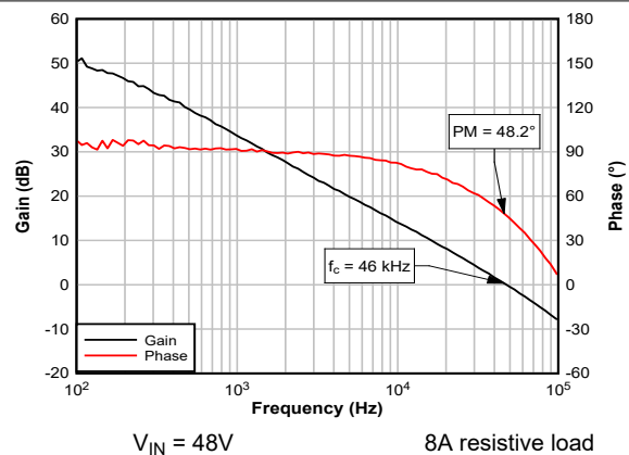
图 8-18. Bode Plot, 5V Output
