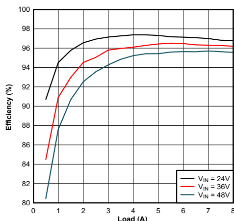
典型效率, V_{OUT} = 12V , f_{SW} = 400kHz
