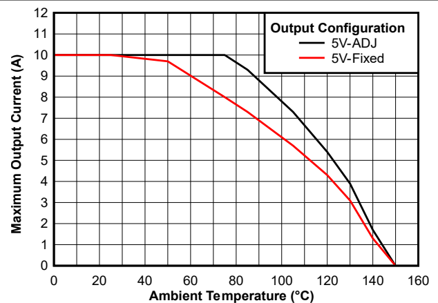
图 7-7. 最大输出电流与环境温度间的关系
