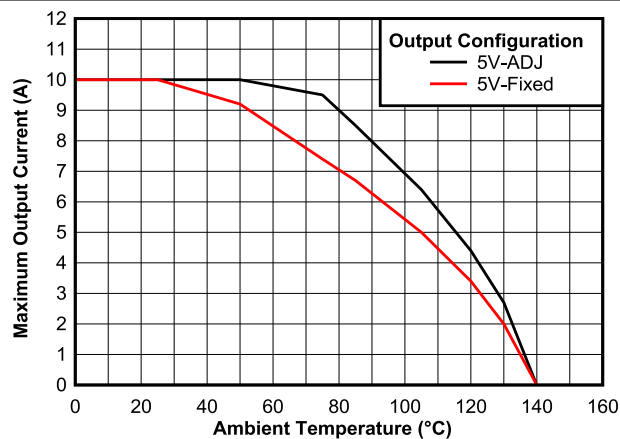
图 7-6. 最大输出电流与环境温度间的关系
