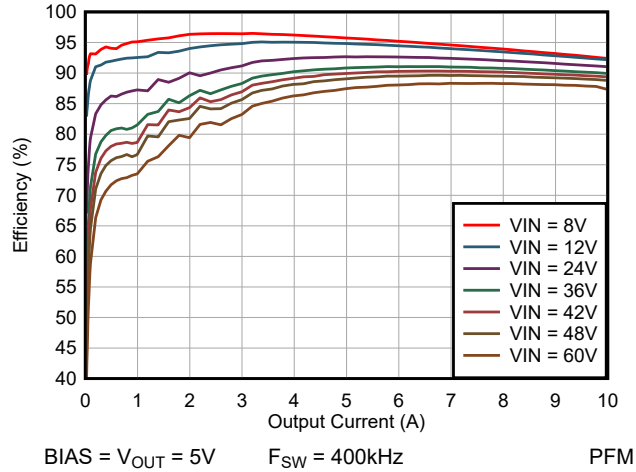
图 5-7. 效率与 I_{OUT} 之间的关系, 线性标度
